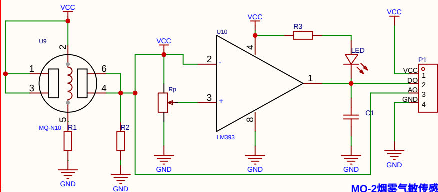
MQ-2烟雾气敏传感器
