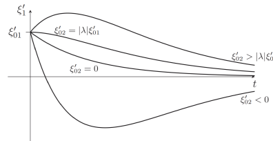
Abbildung 13.25: Zeitverlauf für den aperiodisch gedämpften Fall
