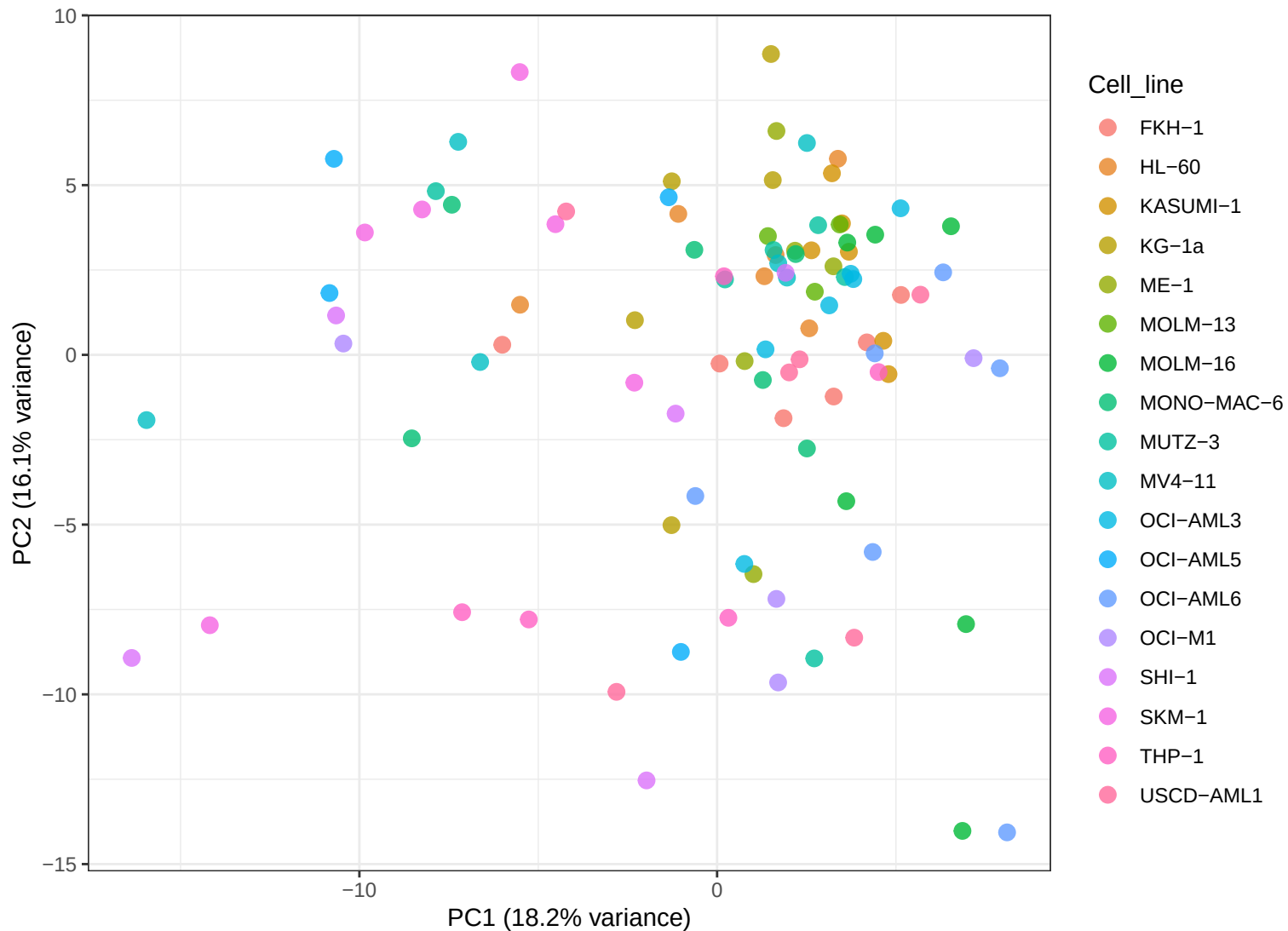
PCA - hPTM
