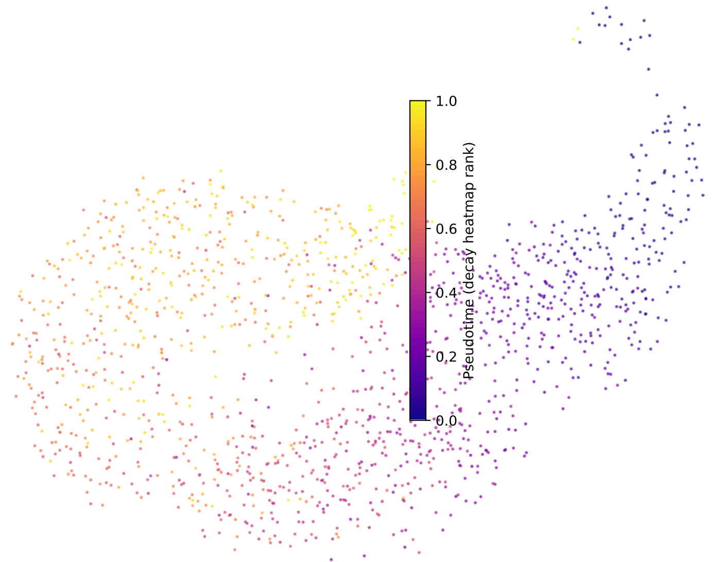
UMAP
