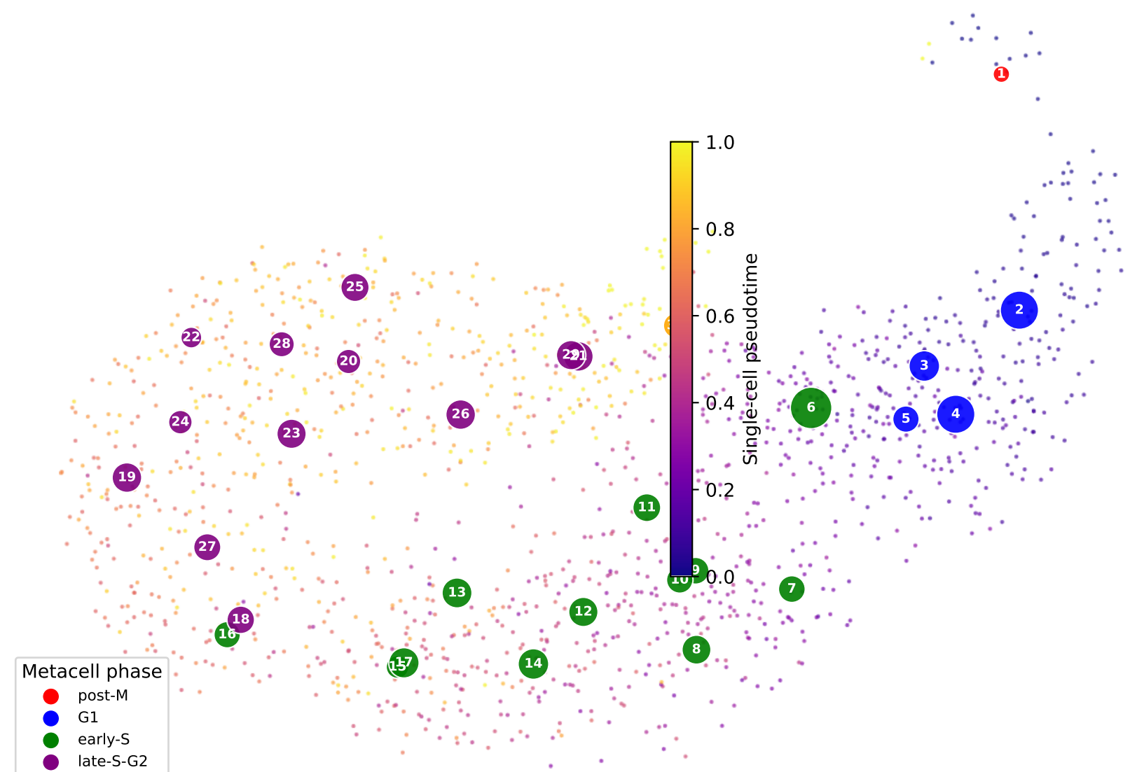
UMAP
