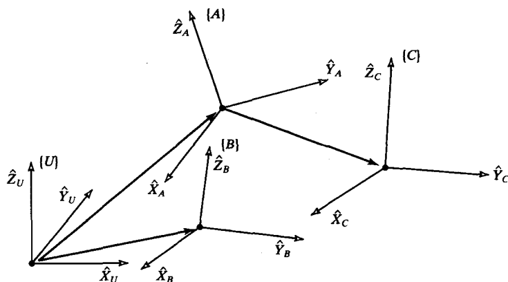
图2-3 几个坐标系举例
