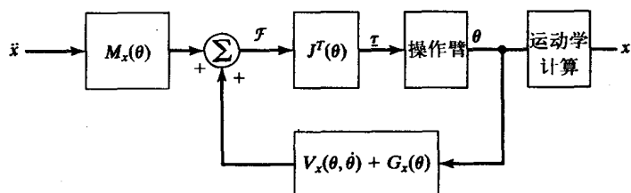
图11-11 第10章中介绍的笛卡儿解耦方案
