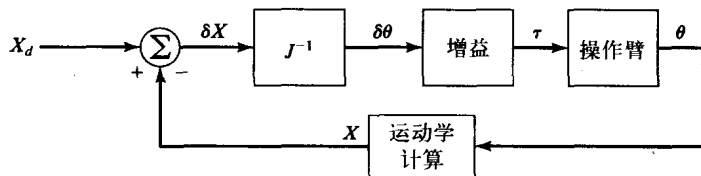
图10-12 逆雅可比笛卡儿空间控制方法
