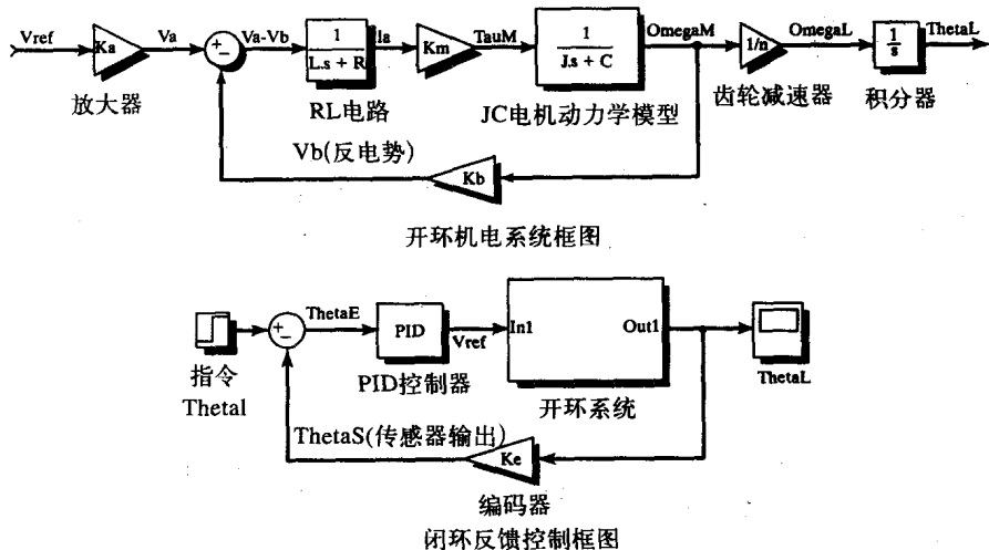
图9-16 由一个直流伺服电机电枢控制器驱动的ARMII电动肩关节/连杆的线性开环系统的动力学模型
