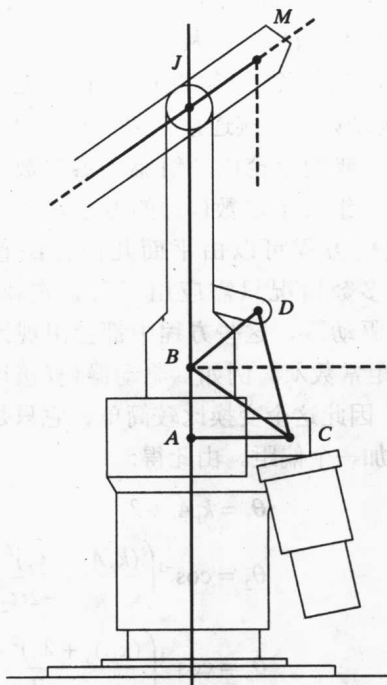
图3-23 Yasukawa驱动器和连杆2的运动示意图
