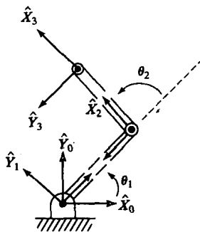
图5-9 两连杆操作臂的坐标系布局
