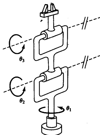
图3-38 三连杆RRR操作臂 (习题3.18)
