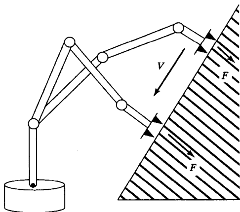
图1-14 为了使操作臂以恒力在一个表面上滑动，必须应用力-位置混合控制系统
