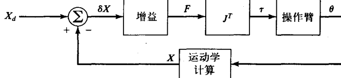
图10-13 转置雅可比笛卡儿空间控制方法
