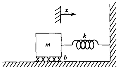
图9-2 具有摩擦的质量-弹簧系统
