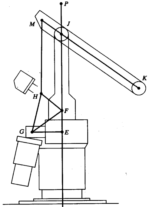
图3-24 Yasukawa驱动器和连杆3的运动示意图
