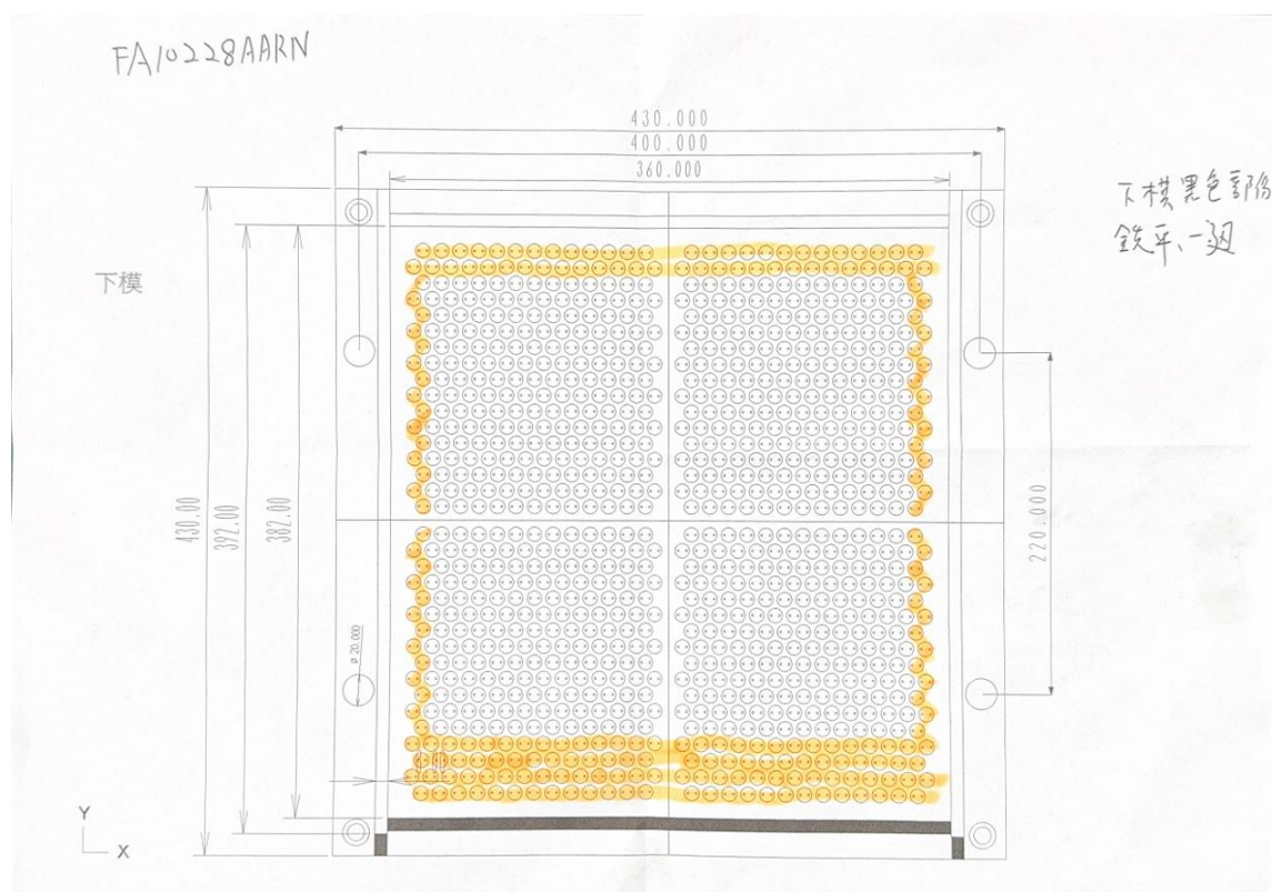
【附件二】模具修改示意图
