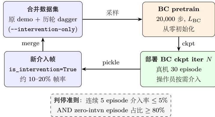
图 6.4: BC + HG-Dagger 迭代工作流。每轮迭代：“训练—部署—介入—合并”四步闭环。(1) 从合并数据集（原 demo + 历轮 dagger， --intervention-only 让原 demo 全保留、dagger 仅取介入帧）随机采样 batch，从零初始化新策略训 BC pretrain 20,000 步;(2) 加载新 ckpt 部署到真机执行 30 episode;(3) 操作员按需介入，所有 transition 写入 pickle 带 is_intervention 标签;(4) 介入帧合并入数据集触发下一轮重训。判停准则同时要求介入率与 zero-intvn 占比满足阈值；真机实测 1-3 轮即可让 pickup 类任务进入稳态。
