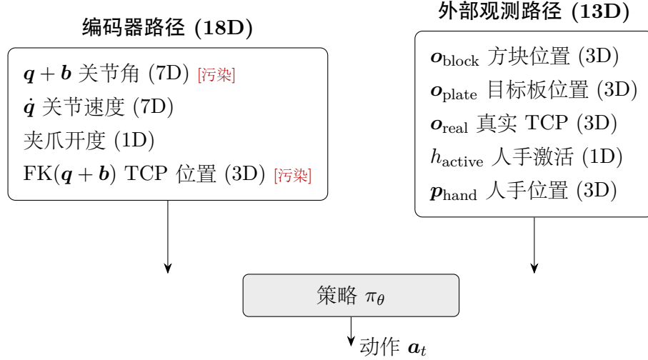
图 4.1: 31 维观测空间的信息通路示意。编码器路径（左，18D）中的关节角与由其导出的 TCP 位置被偏差 b 污染，关节速度与夹爪开度不受影响；外部观测路径（右，13D）包含方块、目标板、独立 TCP 与人手信息，全部与编码器解耦。两路信号在策略网络处汇合，策略原则上可通过 q + b 与 o_{\text{real}} 之间的不一致隐式恢复 b 。
