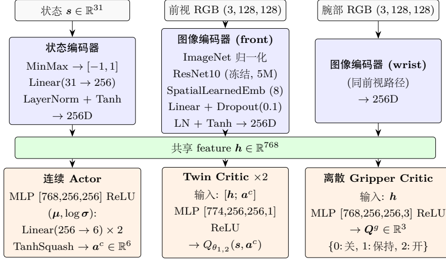
图 4.3: 任务策略的网络架构。三路输入（31 维状态 + 前视/腕部 128 \times 128 RGB）分别经各自的编码器处理后，按通道拼接为 768 维的共享 feature h ；三个头共享 h 作为输入但输出与训练损失各异——连续 Actor 产生 6 维 Cartesian 末端动作、Twin Critic 输出两个标量 Q 值（取最小以抑制高估）、离散 Gripper Critic 输出 3 维 Q 值选择夹爪动作。ResNet10 主干在训练中保持冻结，只更新其后的投影层、状态编码器与三个头。
