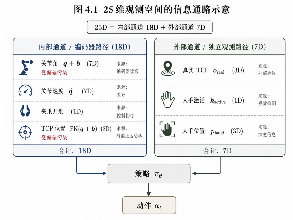
图 4.1: 25 维观测空间的信息通路示意。编码器路径（左，18D）中的关节角与由其导出的 TCP 位置被偏差 \mathbf{b} 污染，关节速度与夹爪开度不受影响；外部观测路径（右，7D）包含独立 TCP 与人手信息，全部与编码器解耦。两路信号在策略网络处汇合，策略原则上可通过 \mathbf{q} + \mathbf{b} 与 \mathbf{o}_{\text{real}} 之间的不一致隐式恢复 \mathbf{b} 。
