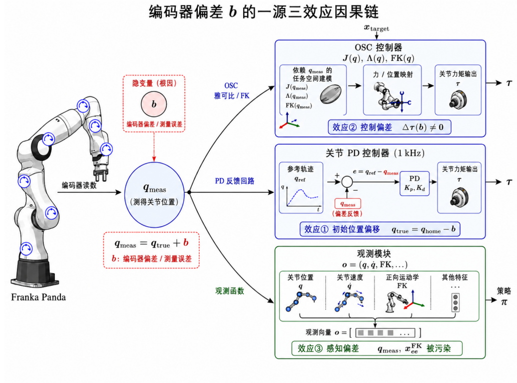
图 3.2: 编码器偏差 b 的因果链: ”一源三效应”结构。单个关节空间隐变量 b 通过三条结构上相互独立的路径——底层 PD 控制器的反馈回路、OSC 控制律中的雅可比与 FK、以及观测函数——同时产生三个可观测的效应。三个效应并非独立故障, 而是同一隐变量在不同模块上的投影。(示意图, 后期将替换为精修版本。)
