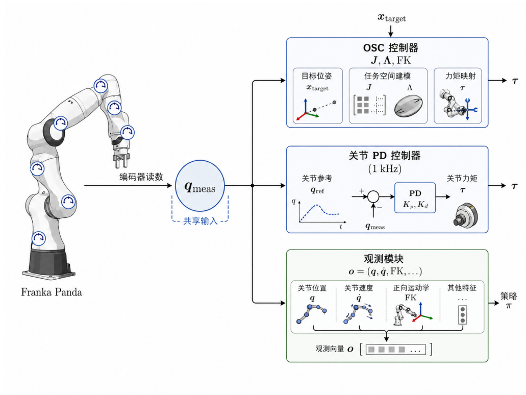
图 3.1: 理想情况下 Franka Panda 的控制与观测数据流。三个下游模块（底层关节 PD、任务层 OSC、观测模块）均以同一个编码器读数 q_{\text{measured}} 作为输入。这一共享依赖是编码器偏差能够同时污染控制与观测的结构性问题。（示意图，后期将替换为精修版本。）
