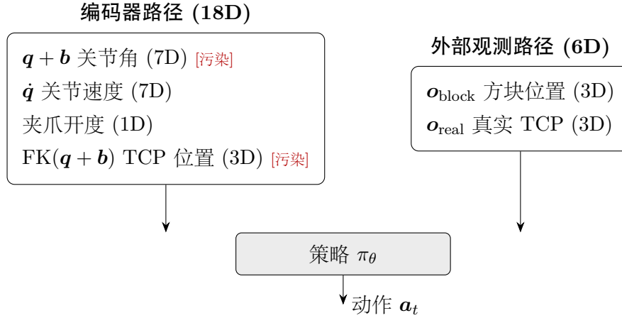
图 4.1: 24 维观测空间的信息通路示意。编码器路径（左）中的关节角与由其导出的 TCP 位置被偏差 \mathbf{b} 污染，关节速度与夹爪开度不受影响；外部观测路径（右）与编码器完全解耦。两路信号在策略网络处汇合，策略原则上可通过两者之间的不一致隐式恢复 \mathbf{b} 。
