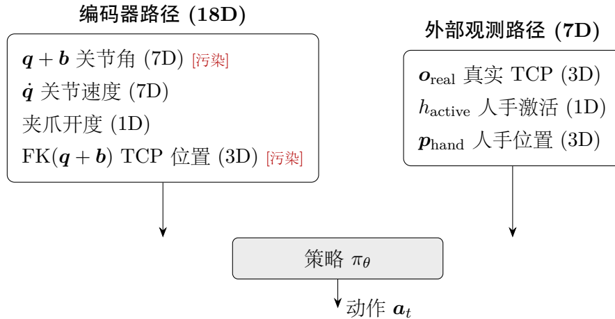
图 4.1: 25 维观测空间的信息通路示意。编码器路径（左，18D）中的关节角与由其导出的 TCP 位置被偏差 \mathbf{b} 污染，关节速度与夹爪开度不受影响；外部观测路径（右，7D）包含独立 TCP 与人手信息，全部与编码器解耦。两路信号在策略网络处汇合，策略原则上可通过 \mathbf{q} + \mathbf{b} 与 \mathbf{o}_{\text{real}} 之间的不一致隐式恢复 \mathbf{b} 。
