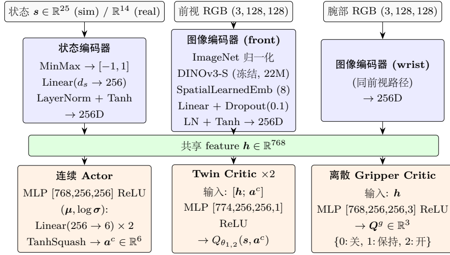
图 4.6: 任务策略的网络架构。三路输入（仿真 25 维 / 真机 14 维状态 + 前视、腕部 128 \times 128 RGB）分别经各自的编码器处理后，按通道拼接为 768 维的共享 feature h ；三个头共享 h 作为输入但输出与训练损失各异——连续 Actor 产生 6 维 Cartesian 末端动作、Twin Critic 输出两个标量 Q 值（取最小以抑制高估）、离散 Gripper Critic 输出 3 维 Q 值选择夹爪动作。DINOv3-S 主干在训练中保持冻结，只更新其后的投影层、状态编码器与三个头。仿真 HIL-SERL 训练四个头的损失，真机 BC 阶段仅训练连续 Actor（critic 与温度参数作为 ckpt schema 占位）。
