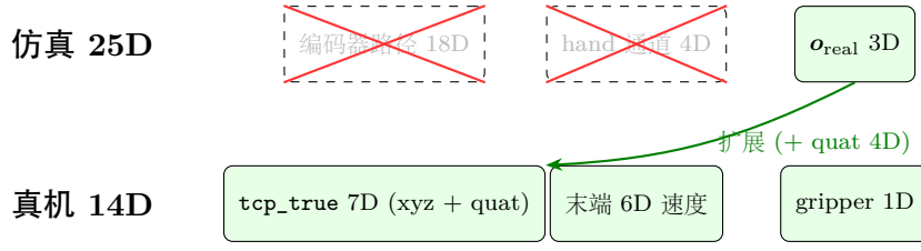
图 4.3: 真机 14 维观测与仿真 25 维 (图 4.1) 的通路差异。仿真侧编码器路径 18D ( \mathbf{q} + \mathbf{b} 、 \dot{\mathbf{q}} 、夹爪开度、 \text{FK}(\mathbf{q} + \mathbf{b}) ) 与 hand 通道 4D ( h_{\text{active}} 、 \mathbf{p}_{\text{hand}} ) 在真机暂不进观测 (红色叉号); 仅 \mathbf{o}_{\text{real}} 通路保留并扩展为含四元数的 7D 真实 TCP 位姿 ( tcp_true ), 加末端 6D 速度 (线速度 + 角速度, 由 \mathbf{J}(\mathbf{q}) \cdot \dot{\mathbf{q}} 算得) 与夹爪开度构成 14D。 \mathbf{o}_{\text{real}} 即 Proposition 3.2 中已被仿真验证的”成功信号路径”, 由第七章的 ArUco 外部独立通道提供。
