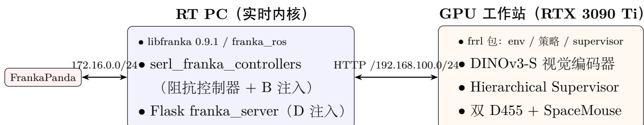
图 6.1: 真机双机架构。RT PC 通过直连以太网与 Franka 控制柜通讯, 运行 1 kHz 实时控制栈; GPU 工作站经独立子网与 RT PC 通讯, 承担策略推理、视觉感知与训练。两机解耦使 GPU 侧策略迭代与 RT PC 侧实时控制独立演进。
