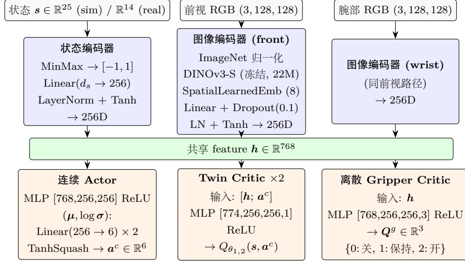
图 4.2: 任务策略的网络架构。三路输入（仿真 25 维 / 真机 14 维状态 + 前视、腕部 128 \times 128 RGB）分别经各自的编码器处理后，按通道拼接为 768 维的共享 feature h ；三个头共享 h 作为输入但输出与训练损失各异——连续 Actor 产生 6 维 Cartesian 末端动作、Twin Critic 输出两个标量 Q 值（取最小以抑制高估）、离散 Gripper Critic 输出 3 维 Q 值选择夹爪动作。DINOv3-S 主干在训练中保持冻结，只更新其后的投影层、状态编码器与三个头。仿真 HIL-SERL 训练四个头的损失，真机 BC 阶段仅训练连续 Actor（critic 与温度参数作为 ckpt schema 占位）。
