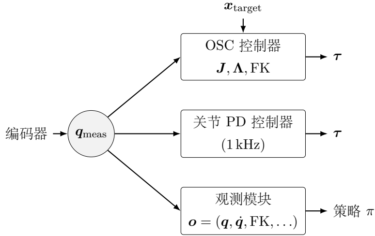
图 3.1: 理想情况下 Franka Panda 的控制与观测数据流。三个下游模块（底层关节 PD、任务层 OSC、观测模块）均以同一个编码器读数 q_{\text{measured}} 作为输入。这一共享依赖是编码器偏差能够同时污染控制与观测的结构性原因。（示意图，后期将替换为精修版本。）
