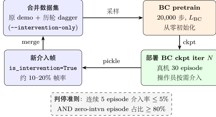
图 6.4: BC + HG-Dagger 迭代工作流程。每轮迭代：“训练—部署—介入—合并”四步闭环。(1) 从合并数据集（原 demo + 历轮 dagger, --intervention-only 让原 demo 全保留、dagger 仅取介入帧）随机采样 batch，从零初始化新策略训 BC pretrain 20,000 步；(2) 加载新 ckpt 部署到真机执行 30 episode；(3) 操作员按需介入，所有 transition 写入 pickle 带 is_intervention 标签；(4) 介入帧合并入数据集触发下一轮重训。判停准则同时要求介入率与 zero-intvn 占比满足阈值；真机实测 1-3 轮即可让 pickup 类任务进入稳态。
