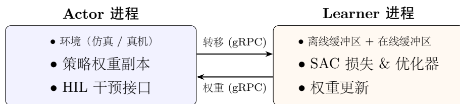
图 5.1: HIL-SERL 的 Actor-Learner 分布式架构。Actor 负责与环境交互、接收 HIL 干预、写入在线缓冲区；Learner 持有缓冲区与优化器，负责混合采样、SAC 更新并回推权重。两侧通过 gRPC 通讯，环境采样与梯度更新完全解耦。
