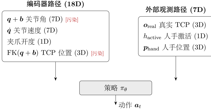
图 4.1: 25 维观测空间的信息通路示意。编码器路径（左，18D）中的关节角与由其导出的 TCP 位置被偏差 b 污染，关节速度与夹爪开度不受影响；外部观测路径（右，7D）包含独立 TCP 与人手信息，全部与编码器解耦。两路信号在策略网络处汇合，策略原则上可通过 q + b 与 o_{\text{real}} 之间的不一致隐式恢复 b 。
