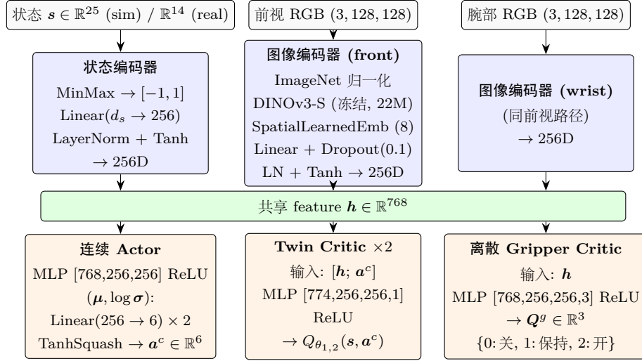
图 4.2: 任务策略的网络架构。三路输入（仿真 25 维 / 真机 14 维状态 + 前视、腕部 128 \times 128 RGB）分别经各自的编码器处理后，按通道拼接为 768 维的共享 feature h ；三个头共享 h 作为输入但输出与训练损失各异——连续 Actor 产生 6 维 Cartesian 末端动作、Twin Critic 输出两个标量 Q 值（取最小以抑制高估）、离散 Gripper Critic 输出 3 维 Q 值选择夹爪动作。DINOv3-S 主干在训练中保持冻结，只更新其后的投影层、状态编码器与三个头。仿真 HIL-SERL 训练四个头的损失，真机 BC 阶段仅训练连续 Actor（critic 与温度参数作为 ckpt schema 占位）。
