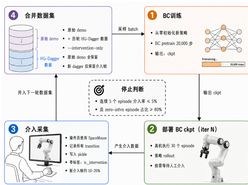
图 6.4: BC + HG-Dagger 迭代工作流程。每轮迭代：“训练—部署—介入—合并”四步闭环。(1) 从合并数据集（原 demo + 历轮 dagger，--intervention-only 让原 demo 全保留、dagger 仅取介入帧）随机采样 batch，从零初始化新策略训 BC pretrain 20,000 步；(2) 加载新 ckpt 部署到真机执行 30 episode；(3) 操作员按需介入，所有 transition 写入 pickle 带 is_intervention 标签；(4) 介入帧合并入数据集触发下一轮重训。判停准则同时要求介入率与 zero-intvn 占比满足阈值；真机实测 1-3 轮即可让 pickup 类任务进入稳态。
