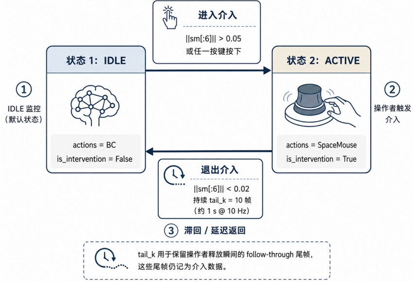
图 6.3: HG-Dagger 介入状态机。IDLE 态下 actions 由 BC 策略生成、不标介入; 推杆量 \|sm[:6]\| > 0.05 或任一按键按下时切到 ACTIVE, actions 改由 SpaceMouse 提供并标为介入; 推杆量 < 0.02 持续 tail\_k = 10 帧 (约 1s @ 10Hz) 后切回 IDLE。tail_k 把“释放瞬间”的 follow-through 帧也保留为介入数据, 捕获恢复尾巴的纠错信号。
