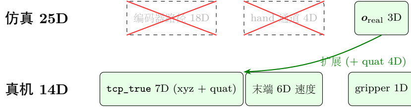
图 6.2: 真机 14 维观测与仿真 25 维 (图 4.1) 的通路差异。仿真侧编码器路径 18D ( \mathbf{q} + \mathbf{b} 、 \dot{\mathbf{q}} 、夹爪开度、 \text{FK}(\mathbf{q} + \mathbf{b}) ) 与 hand 通道 4D ( \mathbf{h}_{\text{active}} 、 \mathbf{p}_{\text{hand}} ) 在真机暂不进观测 (红色叉号); 仅 \mathbf{o}_{\text{real}} 通路保留并扩展为含四元数的 7D 真实 TCP 位姿 ( tcp_true ), 加末端 6D 速度 (线速度 + 角速度, 由 \mathbf{J}(\mathbf{q}) \cdot \dot{\mathbf{q}} 算得) 与夹爪开度构成 14D。 \mathbf{o}_{\text{real}} 即 Proposition 3.2 中已被仿真验证的”成功信号路径”, 由第 6.2.2 节描述的 /getstate_true 外部独立通道提供。
