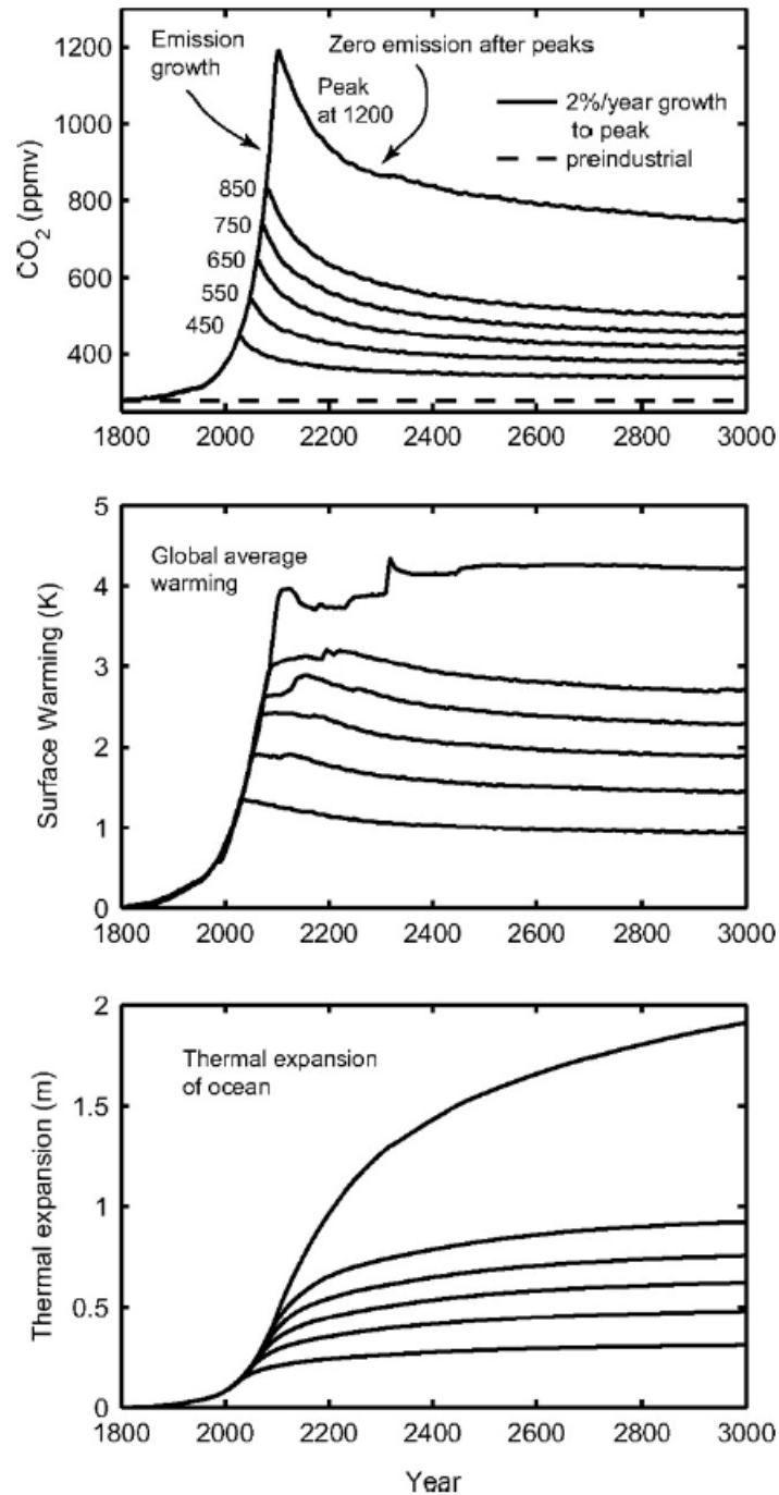
Abbildung 3.11: Kohlendioxid und globale Veränderungen des Klimasystems (im Vergleich zu den vorindustriellen Bedingungen im Jahr 1765). Quelle: Solomon u. a. (2009).
