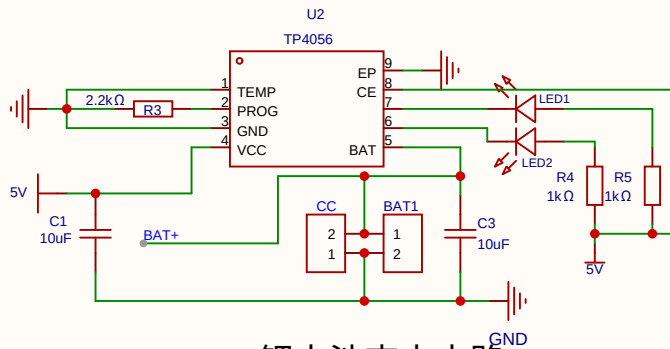
锂电池充电电路
