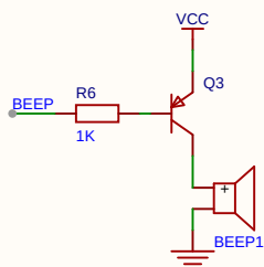
蜂鸣器
