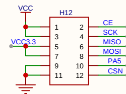
NRF24L01
