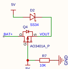
供电切换电路
