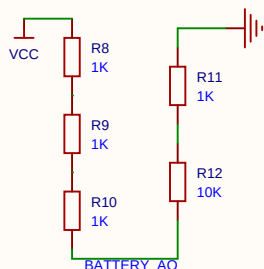
电池电压检测电路
