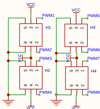
8舵机排插
