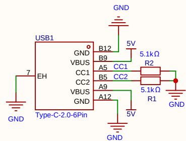
Type-c电路
