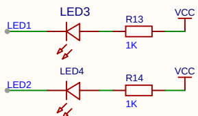
LED电路
