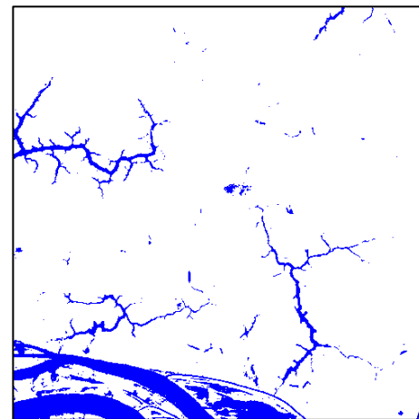
Mahalanobis
