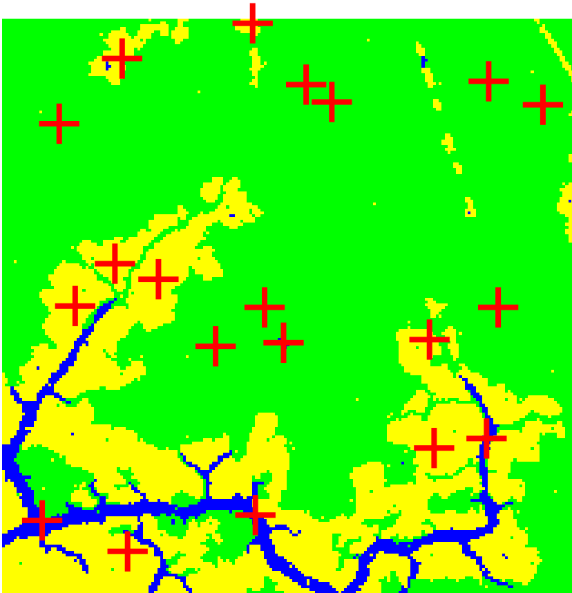
Imagem Classificada
