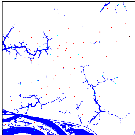
Mínima Distância
