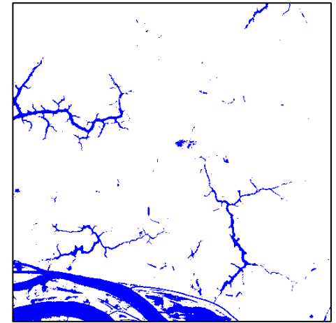
Mahalanobis
