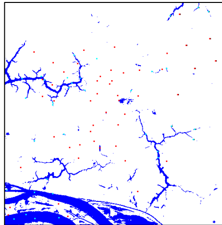
Mahalanobis
