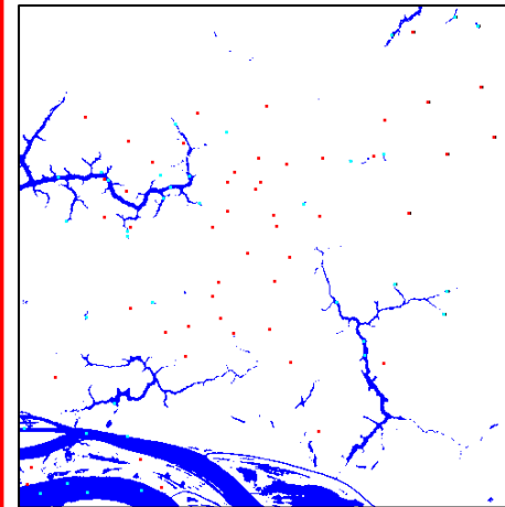
SVM
