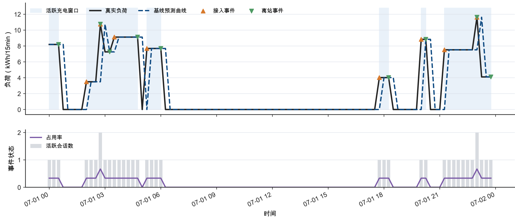
真实负荷、预测曲线与事件窗口
