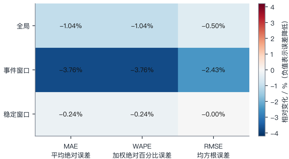
c 本文方法相对强行为基线的指标变化
