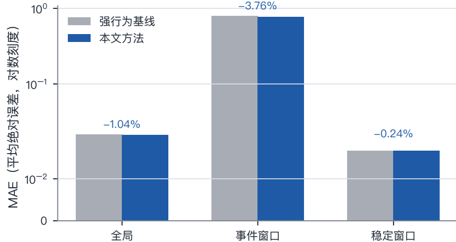
c 本文方法相对强行为基线的指标变化
