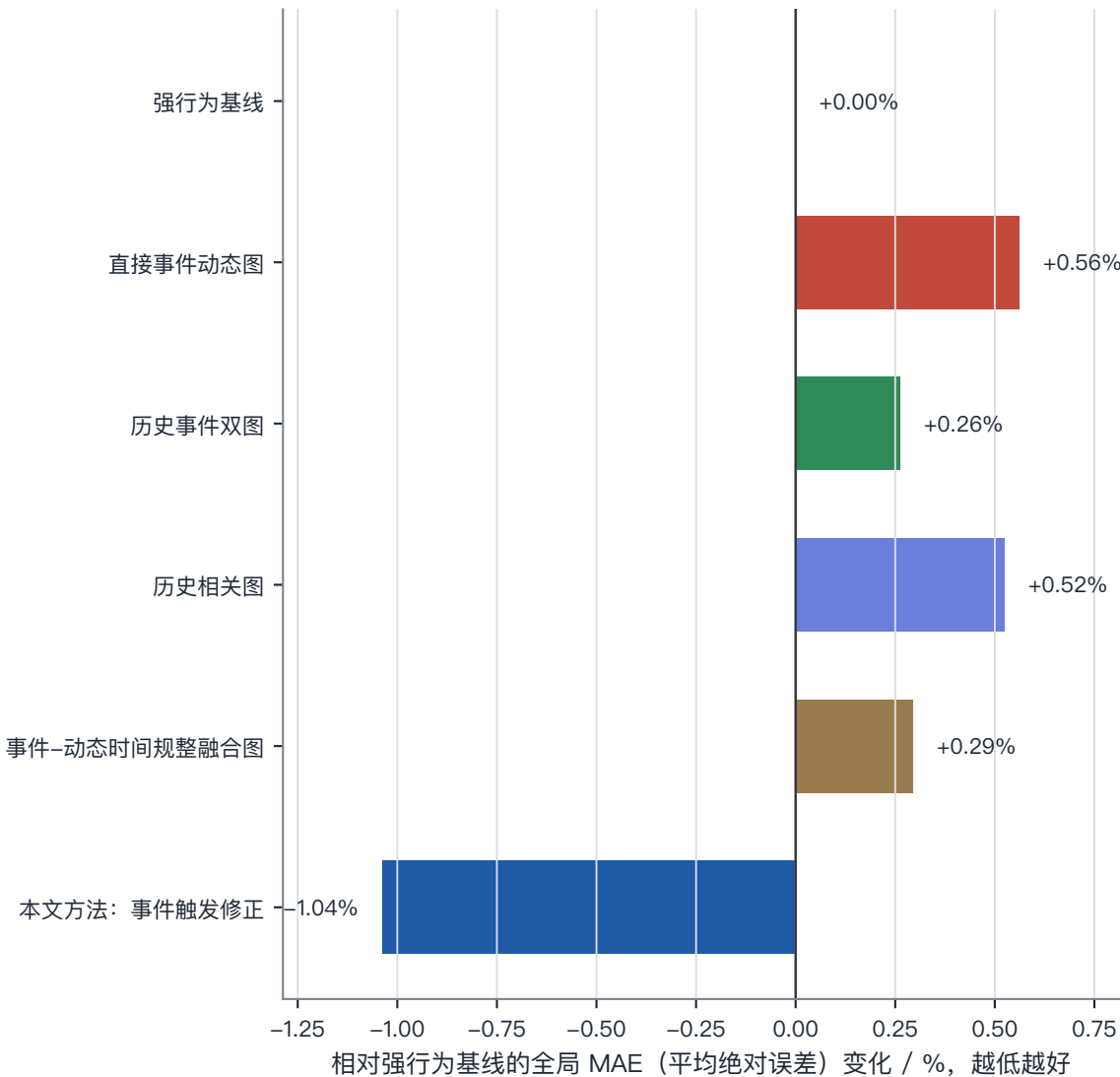
a 全局替换与事件触发修正的对照
