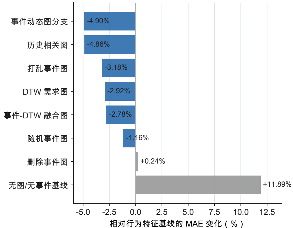
改进来自事件与图结构信息
