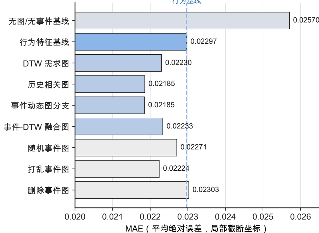
弱基线与图结构分支的同口径对照
