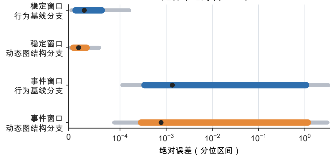
A 逐样本绝对误差分布
