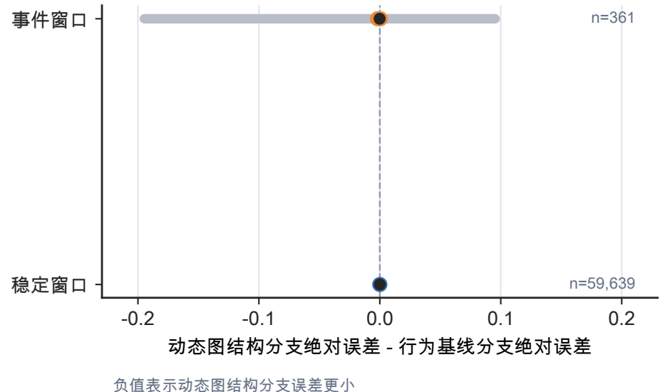
B 成对误差差值分布
