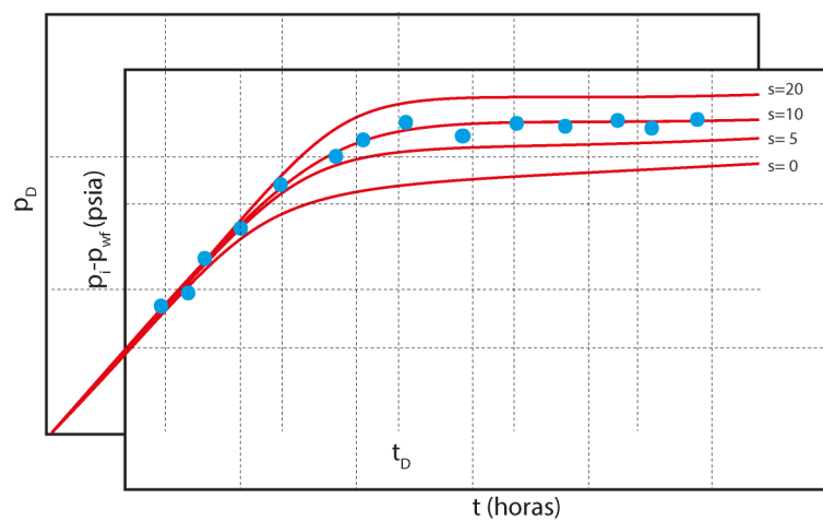
Figura 7.8: Ajuste de los datos de presión registrados con el comportamiento de las curvas tipo de Ramey
