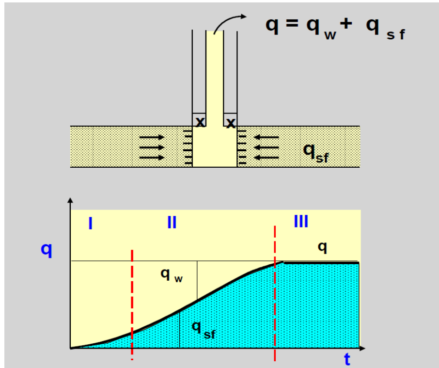
Figura 3.3: Efecto de almacenamiento en el pozo (Cinco-Ley, 1995)
