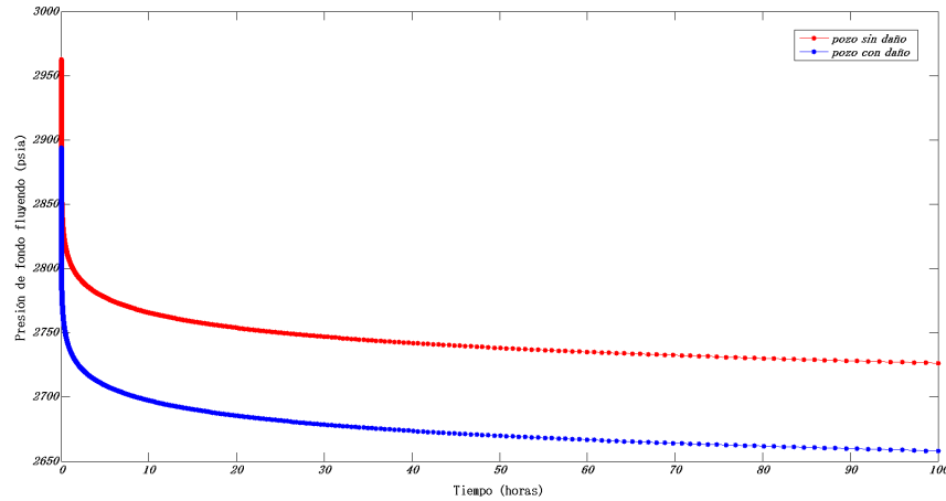
Figura 5.9: Comportamiento de los perfiles de presión en el pozo para ilustrar el efecto de daño en la formación
