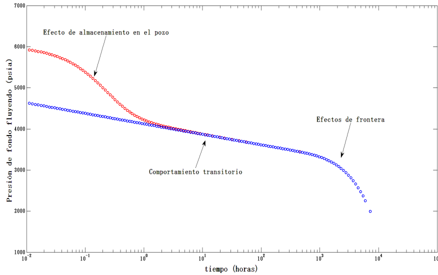
Figura 7.5: Efecto de almacenamiento en un prueba de decremento de presión
