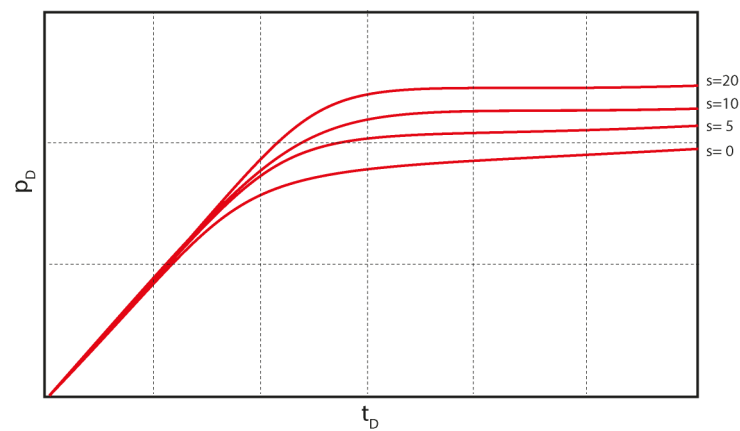
Figura 7.7: Set de curvas tipo de Ramey seleccionado para realizar el ajuste
