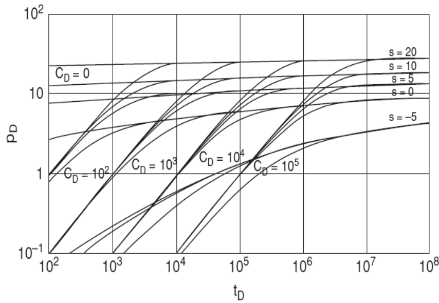
Figura 7.3: Curvas tipo para pruebas de un sólo pozo incluyendo daño y almacenamiento en un yacimiento de comportamiento infinito (Ezekwe, 2010).
