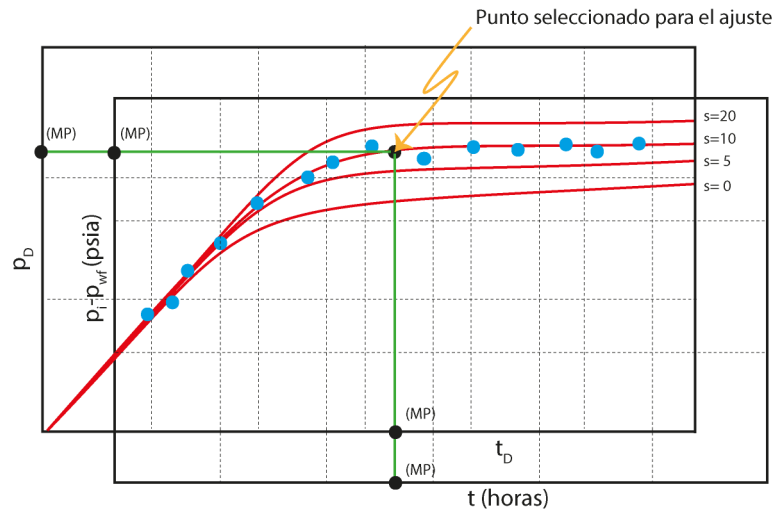
Figura 7.9: Obtención del "Match point"
