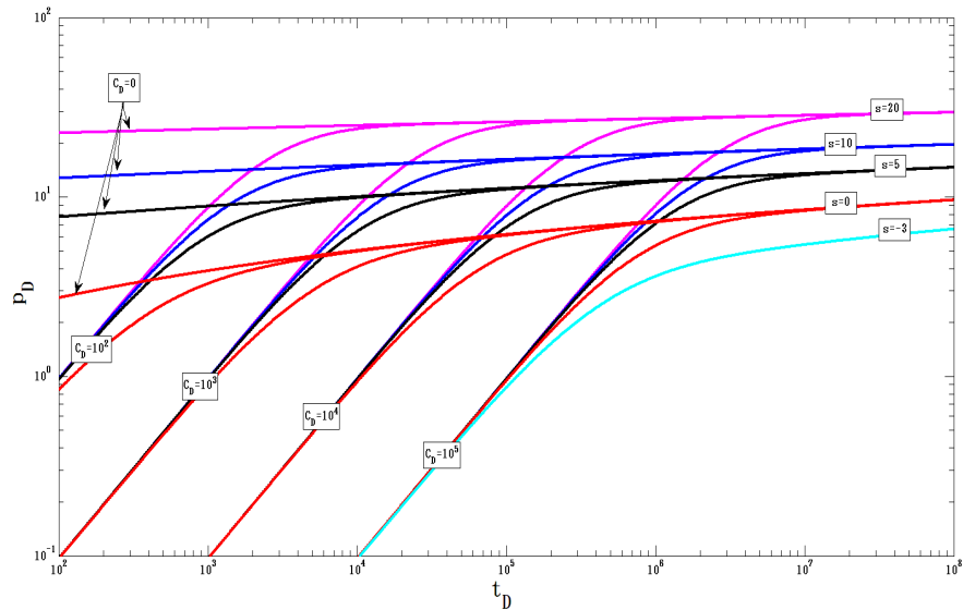
Figura 7.4: Curvas tipo para pruebas de un sólo pozo incluyendo daño y almacenamiento en un yacimiento de comportamiento infinito (Maestría UNAM, 2014)
