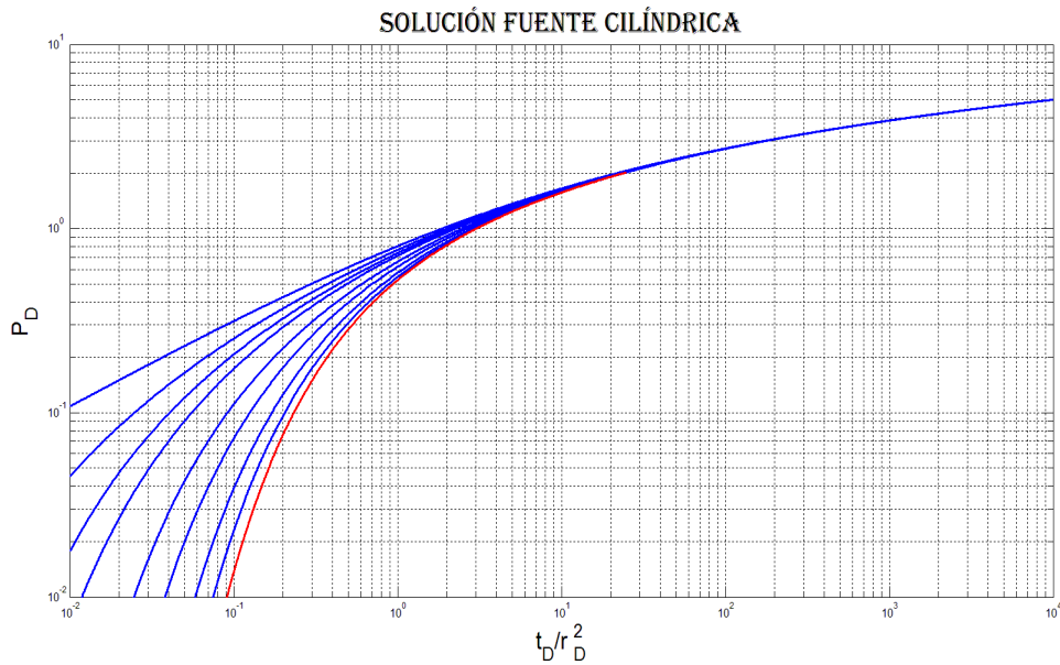
Figura 5.5: Solución exacta y solución línea fuente (Licenciatura, 2013)
