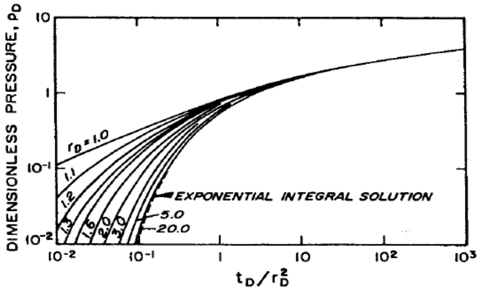
Figura 5.4: Solución exacta y solución línea fuente (Earlougher, 1977)
