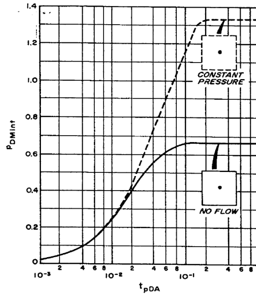
Figura 7.13: Presiones adimensionales de intersección para un pozo colocado en el dentro de un yacimiento cuadrado. (Earlougher, 1977).
