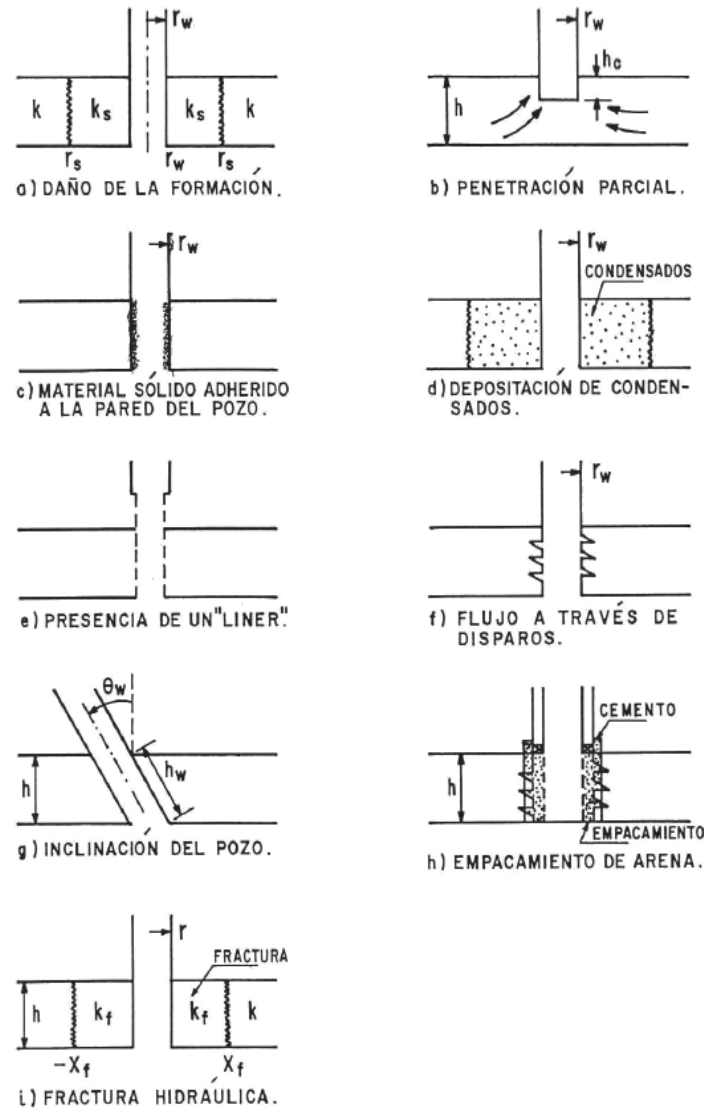
Figura 3.1: Factores que afectan el flujo de fluidos de la formación hacia el pozo (Samaniego, 2012)
