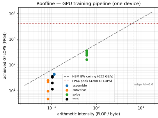
Figura 4: Roofline del pipeline de entrenamiento. Todas las etapas quedan por debajo del techo de cómputo y en la región limitada por ancho de banda.
