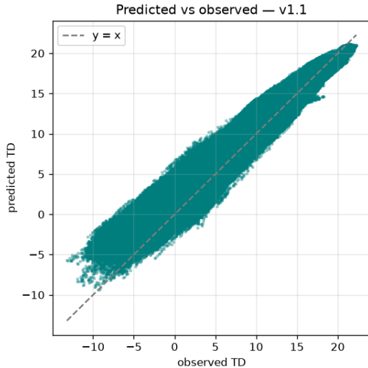
Figura 11: Temperatura de punto de rocío predicha frente a la observada con PISCOt v1.1.
