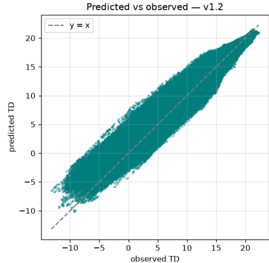
Figura 12: Temperatura de punto de rocío predicha frente a la observada con PISCOt v1.2.
