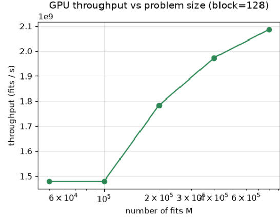
Figura 7: Rendimiento del kernel solve frente a M : la tasa de ajustes por segundo aumenta hasta saturar el dispositivo.
