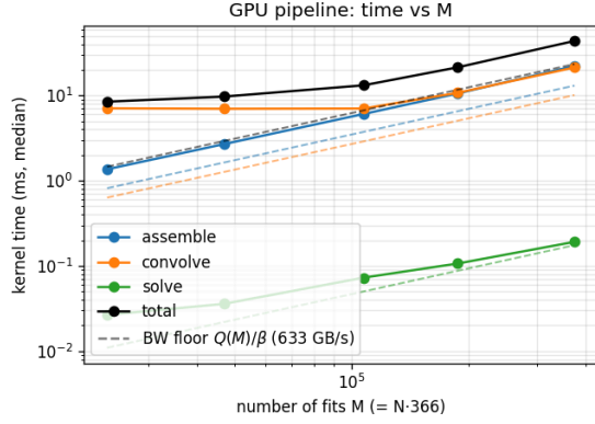
Figura 6: Tiempo de cada etapa frente al tamaño del problema M . Las líneas discontinuas son el piso teórico de ancho de banda T_{\text{bound}}(M) = Q(M)/\beta .
