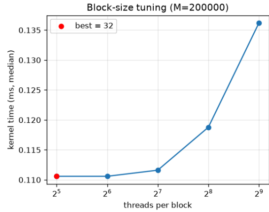
Figura 5: Ajuste del tamaño de bloque del kernel solve ; 32 hilos por bloque fue la mejor configuración en la partición evaluada.
