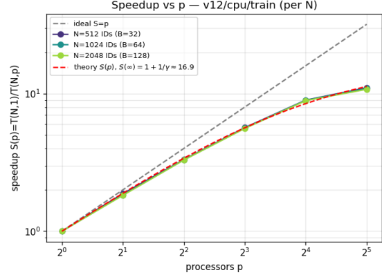
Figura 2: Aceleración observada frente al número de procesos para los tres tamaños de problema.
