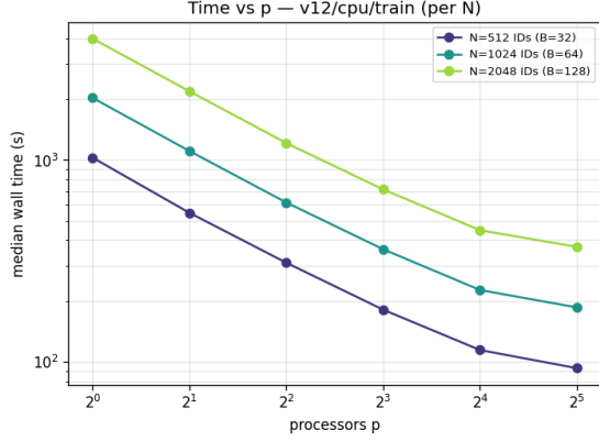
Figura 1: Tiempo de pared del entrenamiento frente al número de procesos para 512, 1024 y 2048 IDs.
