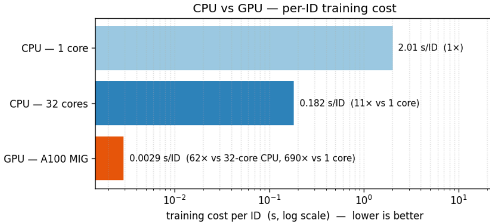
Figura 8: Costo de entrenamiento por ID en escala logarítmica (menor es mejor). La comparación usa el costo por ID porque los benchmarks de CPU y GPU se ejecutaron con tamaños de problema distintos.
