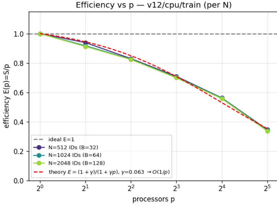
Figura 3: Eficiencia paralela frente al número de procesos. Las curvas de los tres tamaños casi se superponen; la línea roja discontinua representa el modelo de contención de memoria ajustado E(p) = (1 + \gamma)/(1 + \gamma p) .
