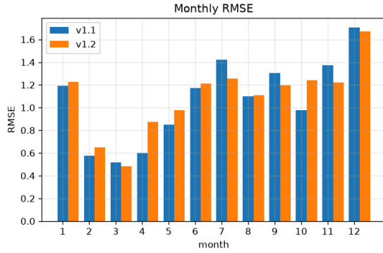
Figura 9: RMSE mensual del pronóstico retenido, PISCOt v1.1 frente a v1.2.
