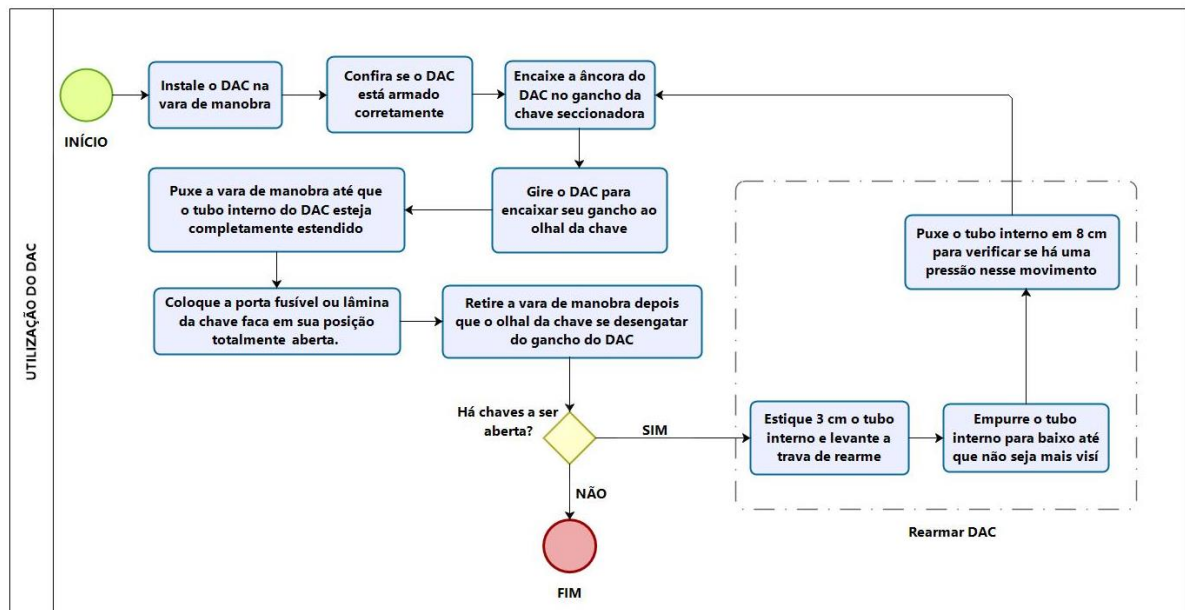
Figura 3 – Fluxograma da utilização do DAC.
