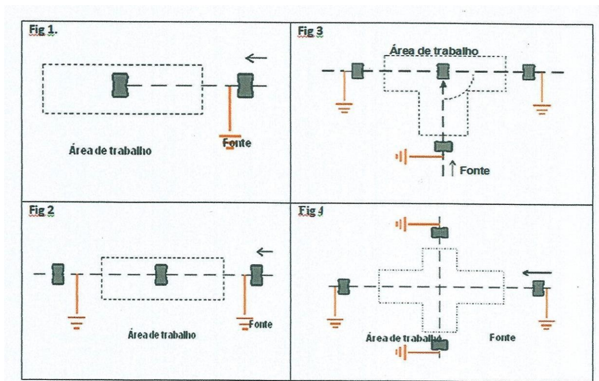
Figura 1 - Trabalho entre pontos de aterramento, exigindo no mínimo dois aterramentos, salvo quando trabalhar no último poste
