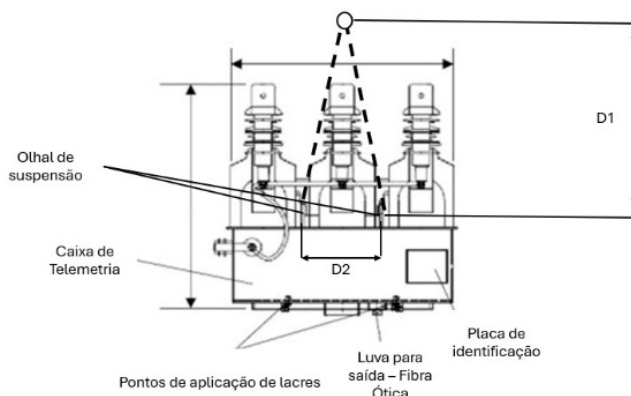
Figura 19 – Comprimento adequado do estropo.
