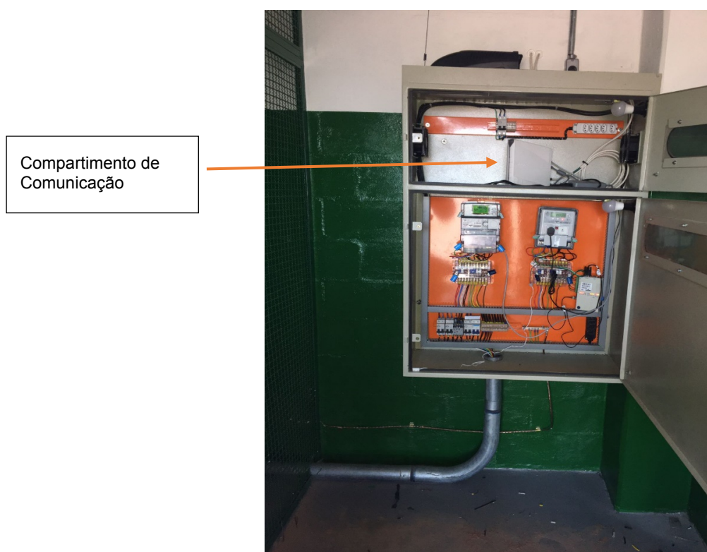
Figura 4 - Painel de Medição – Média tensão
