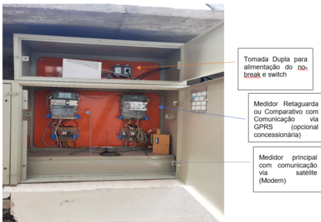
Figura 2 -Painel de medição - baixa tensão 0,6kv
