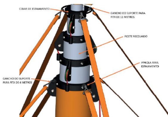
Figura 16 – Pré-instalação das fitas estais
