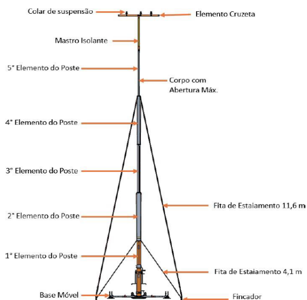
Figura 1 – Poste telescópico do Fabricante Leal – principais componentes
