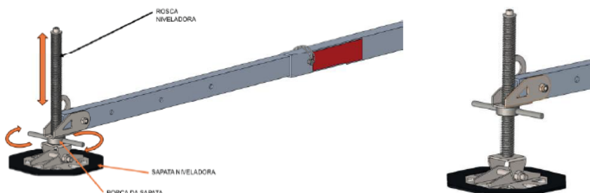
Figura 13 – Nivelamento das sapatas
