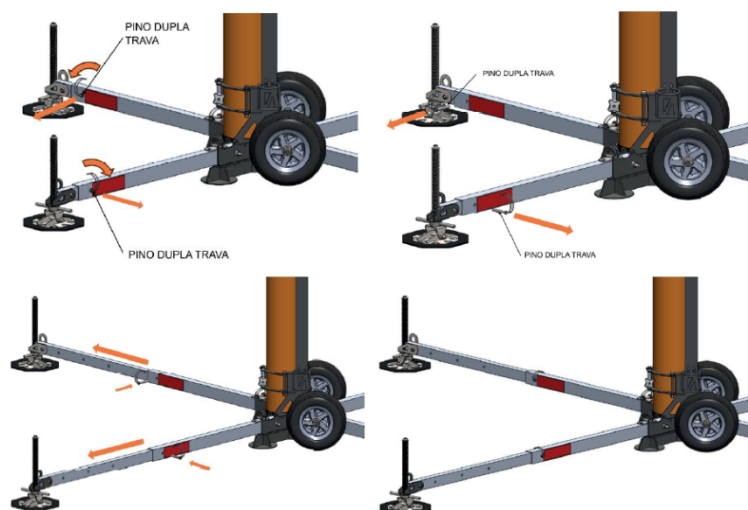
Figura 12 – Extensão das sapatas e inserção dos pinos de travamento
