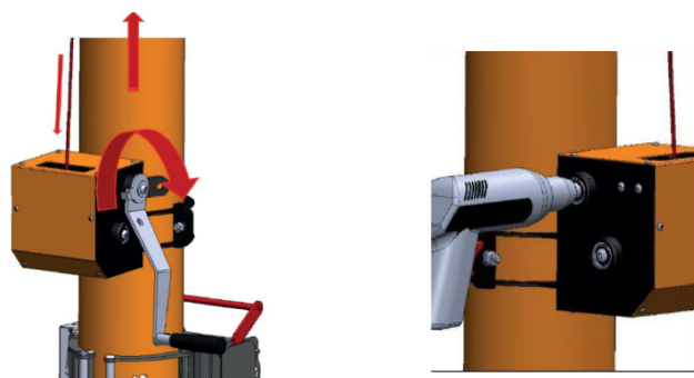
Figura 17 – Modo de subida do poste manual e por parafusadeira, respectivamente
