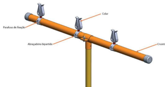
Figura 7 – Instalação do colar para cruzeta
