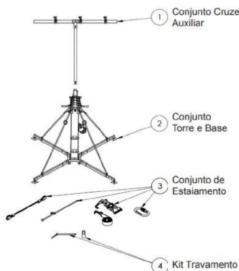
Figura 2 – Modelo do poste telescópico do Fabricante DH
