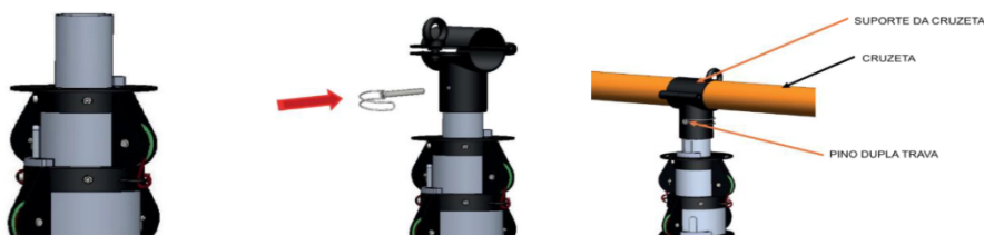
Figura 5 – Instalação do suporte e cruzeta auxiliar
