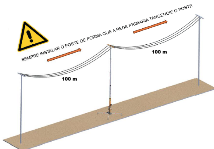
Figura 15 – Distância máxima permitida dos vãos após instalação do poste telescópico
