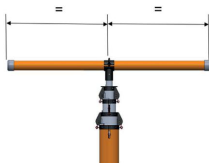
Figura 6 – Posição equidistante da cruzeta auxiliar
