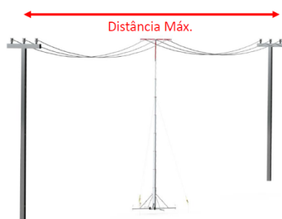
Figura 22 – Distância máxima dos vãos, representação gráfica
