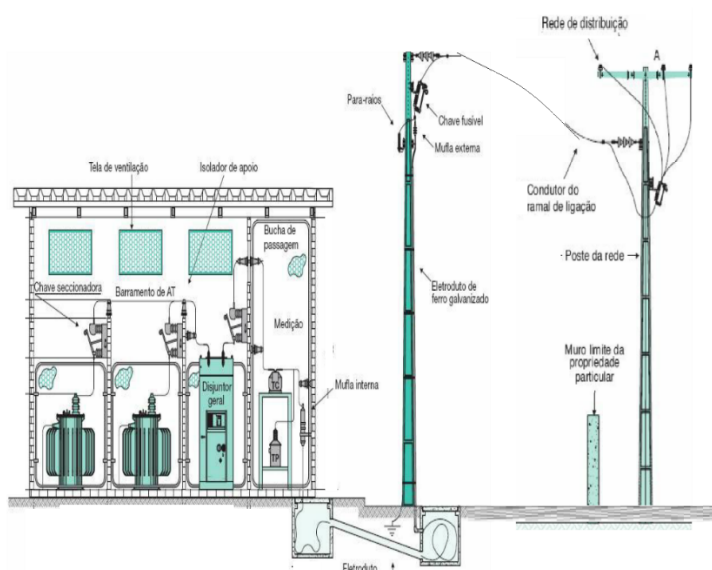
Figura 13 – Subestação do consumidor com entrada subterrânea [Adaptada do livro Instalações Elétricas Industriais]
