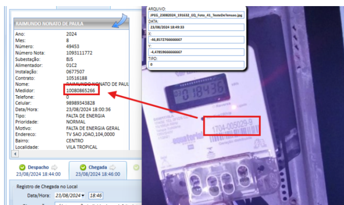
Figura 6 – Exemplo de numeração do medidor divergente da numeração do sistema
