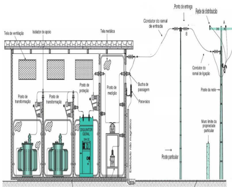
Figura 12 – Subestação do consumidor com entrada aérea [Adaptada do livro Instalações Elétricas Industriais]
