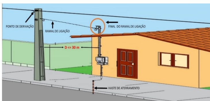
Figura 11 - Final do ramal de ligação em pontalete
