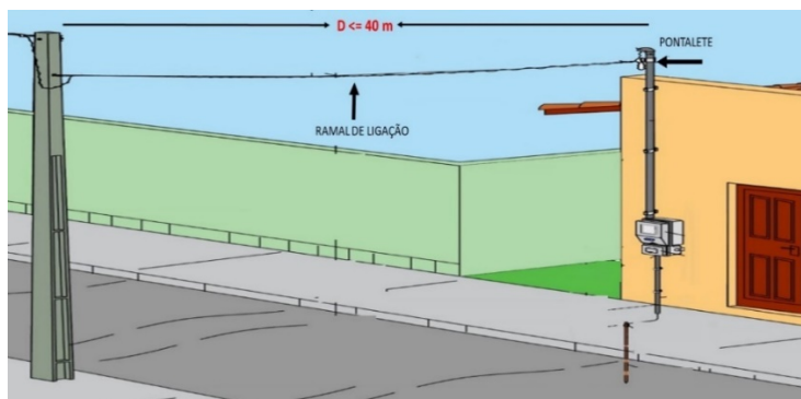
Figura 10 – Entrada de serviço com pontalete do mesmo lado da posteação
