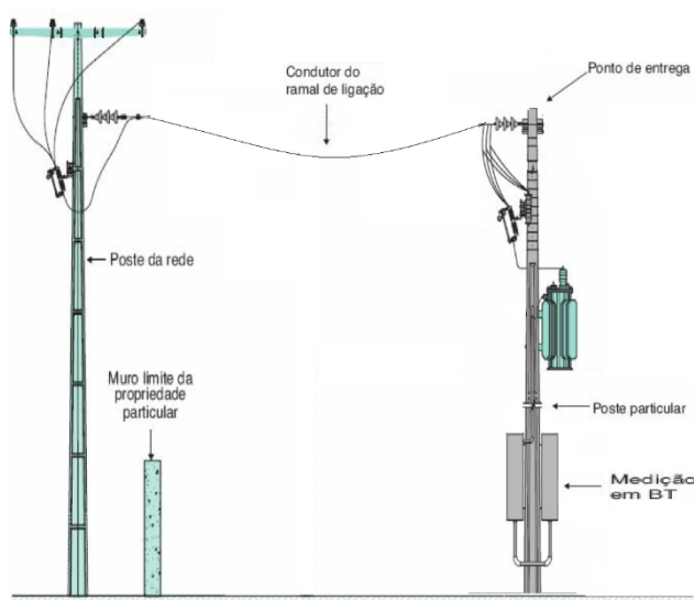
Figura 15 – Subestação do consumidor aérea com medição a BT
