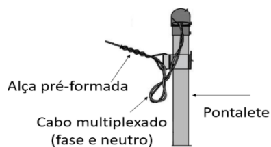
Figura 11 - Final do ramal de ligação em pontalete
