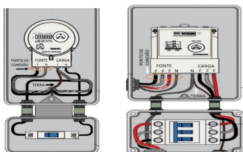
Figura 3 – Modelo de medidor monofásico e trifásico, respectivamente
