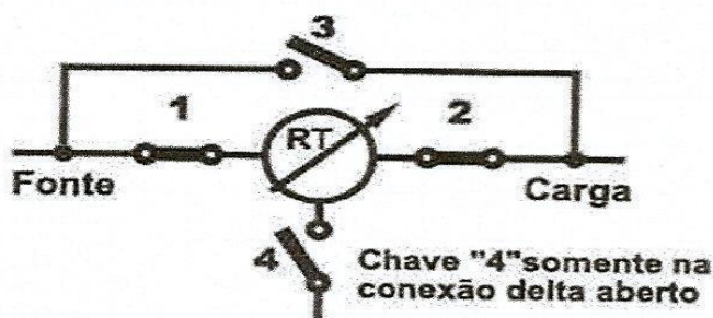
Figura 2 - Chaves Seccionadoras de um Regulador de Tensão Monofásico em Delta Aberto
