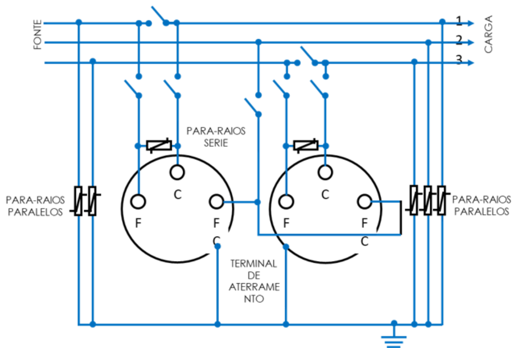
Figura 3 - Chaves Seccionadoras de um Regulador de Tensão em Delta Aberto
