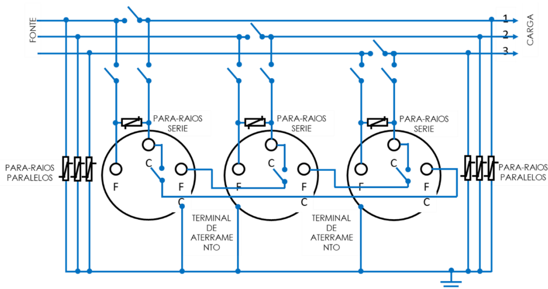
Figura 4 - Chaves Seccionadoras de um Regulador de Tensão Delta Fechado
