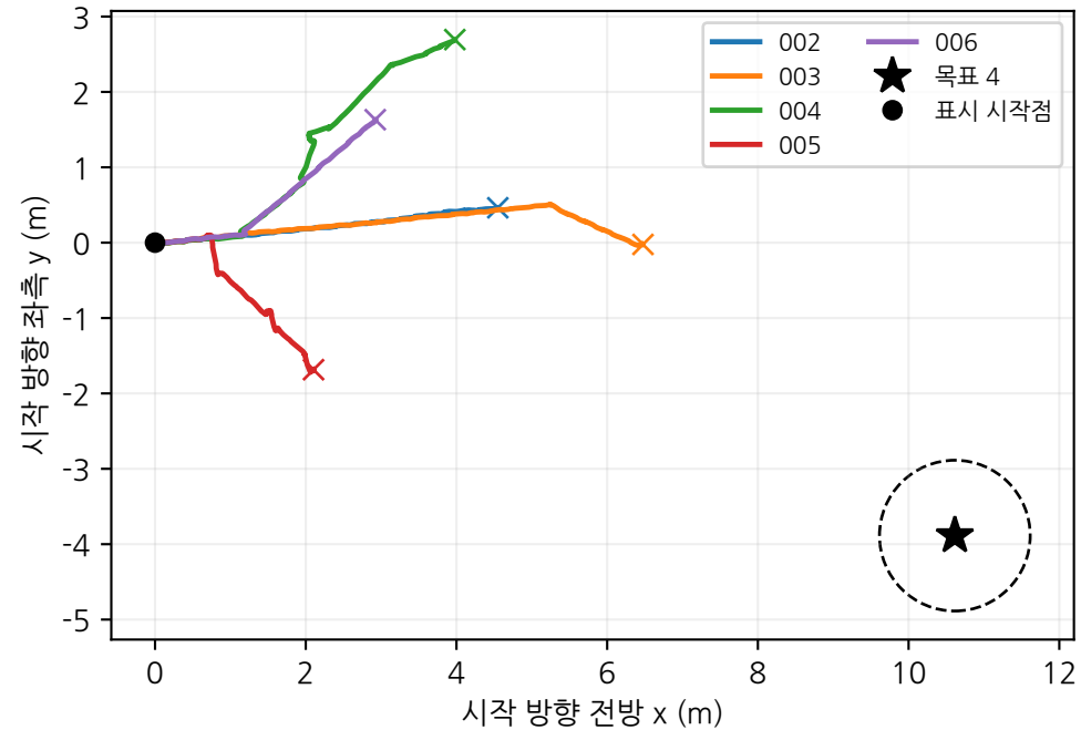
회차별 오도메트리 궤적 · 동일 축척
