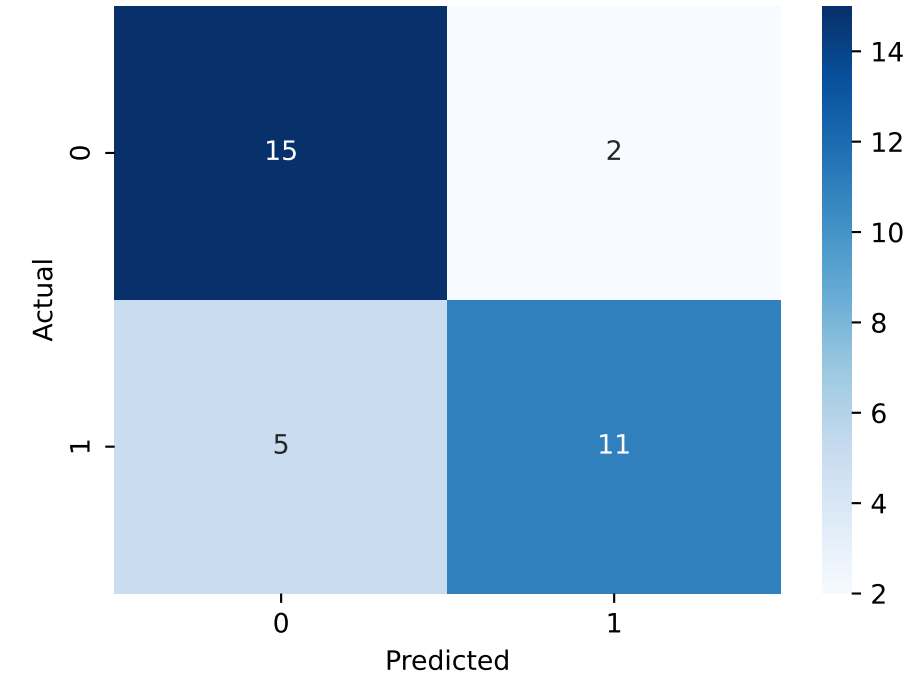
PyTorch Autoencoder
