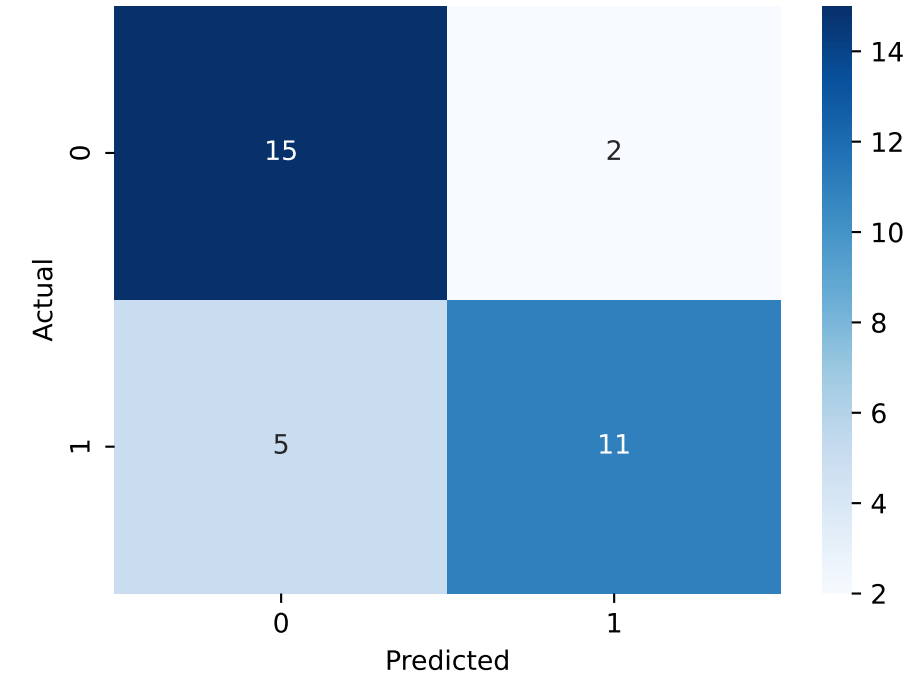
PyTorch Autoencoder
