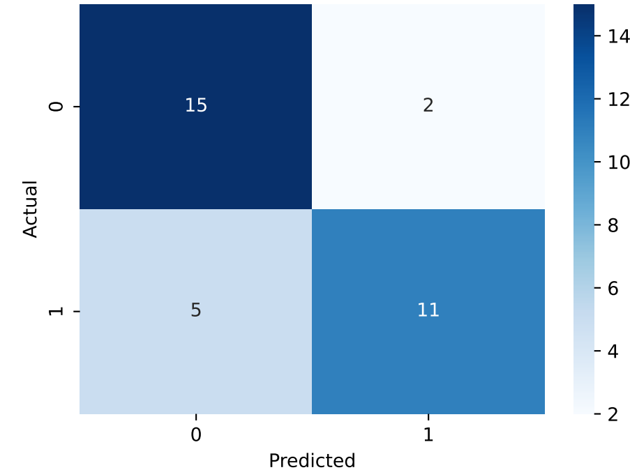
PyTorch Autoencoder
