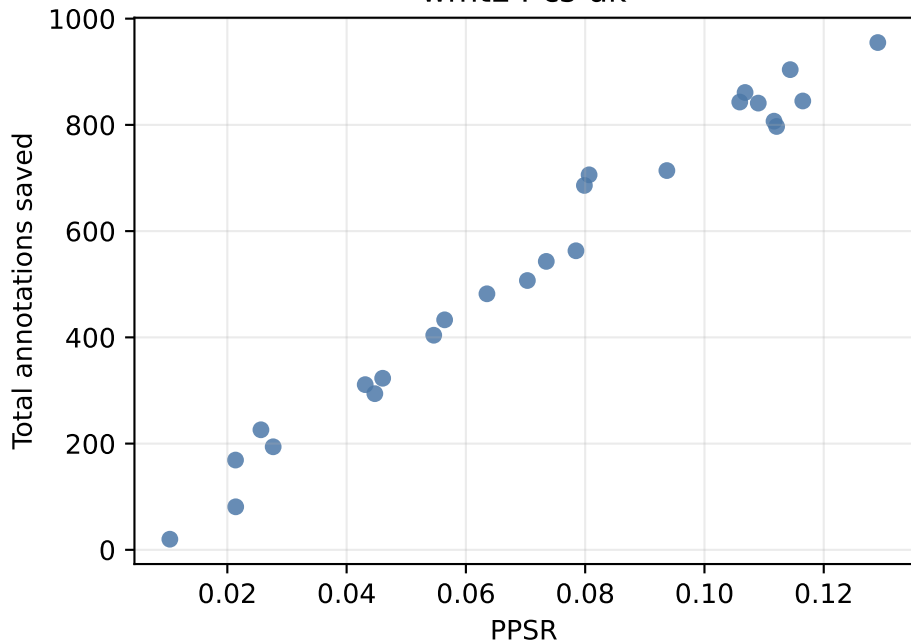
wmt24 cs-uk
