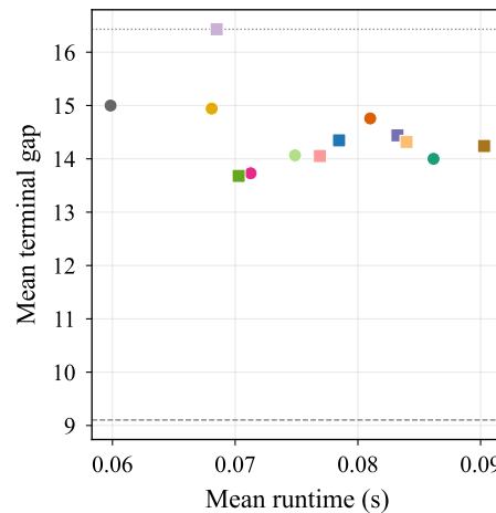
(d) Pareto: gap vs time
