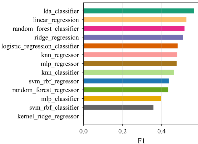
(c) Need-query F1
