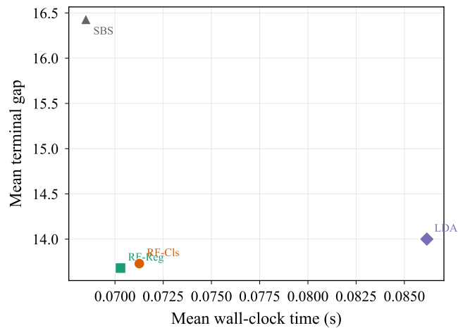
(d) Pareto: gap vs time
