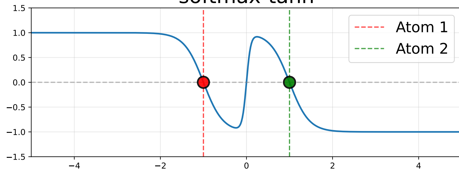
softmax-tanh
