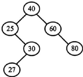
二叉树 T1
