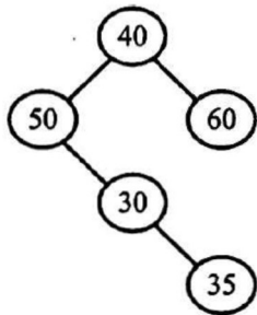
二叉树 T2
