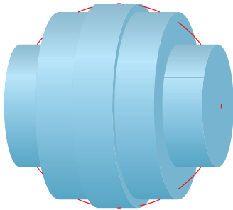
(a) Mediante 5 discos, V \approx 4.2726
