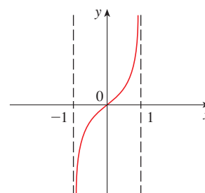
FIGURA 10 y = \tanh^{-1}x dominio = (-1, 1) rango = \mathbb{R}
