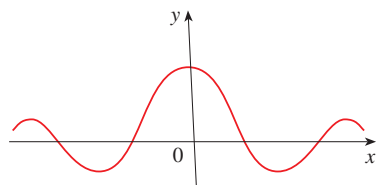
(a) Función par: simetría por reflexión
