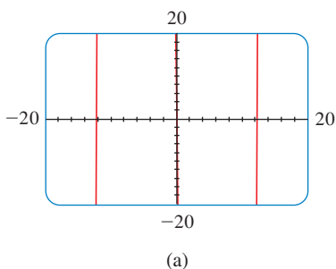
FIGURA 5 y = x^3 - 150x
