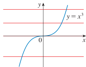
FIGURA 3 f(x) = x^3 es uno a uno
