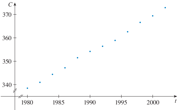
FIGURA 4 Gráfica de dispersión para el nivel de \text{CO}_2
