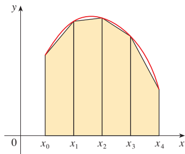
FIGURA 2 Aproximación trapezoidal
