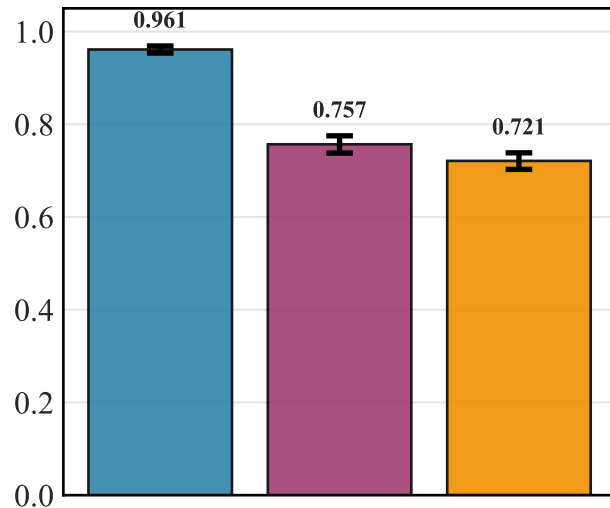
F1 Score
