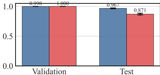
F1 Score
