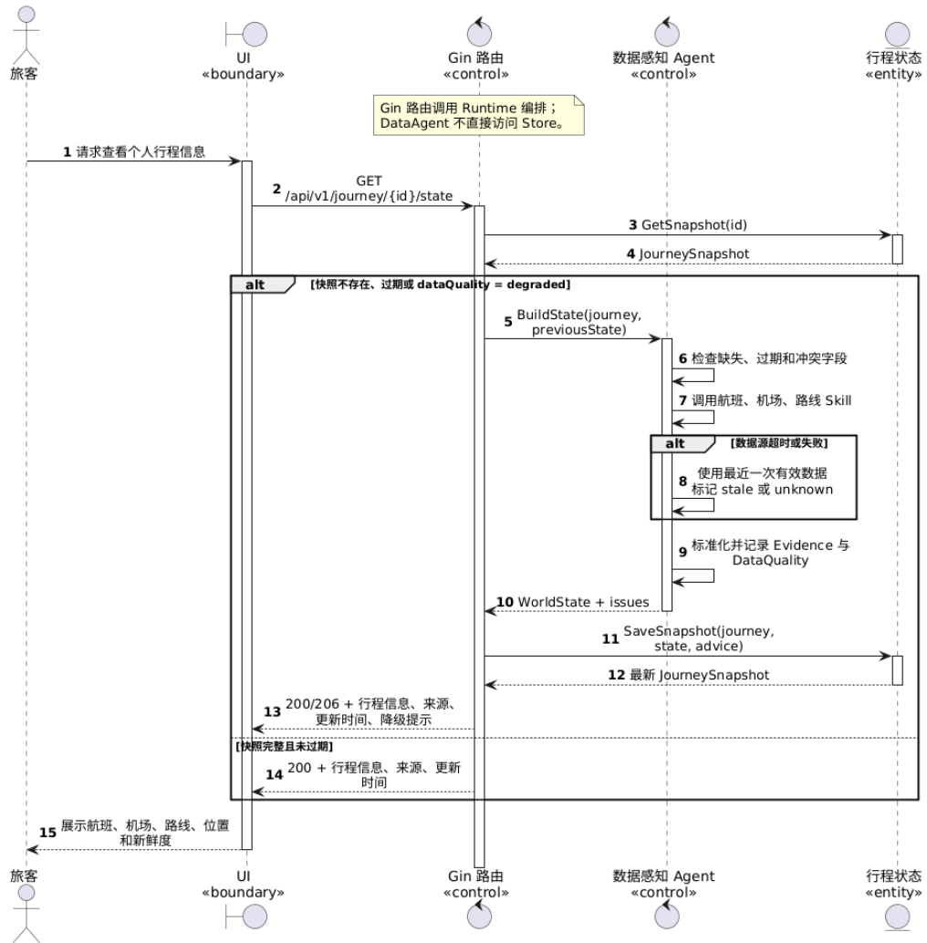
图2-2 系统“获取个人行程信息数据”用例顺序图
