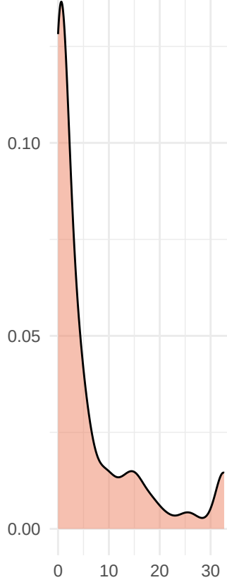
paraquats
