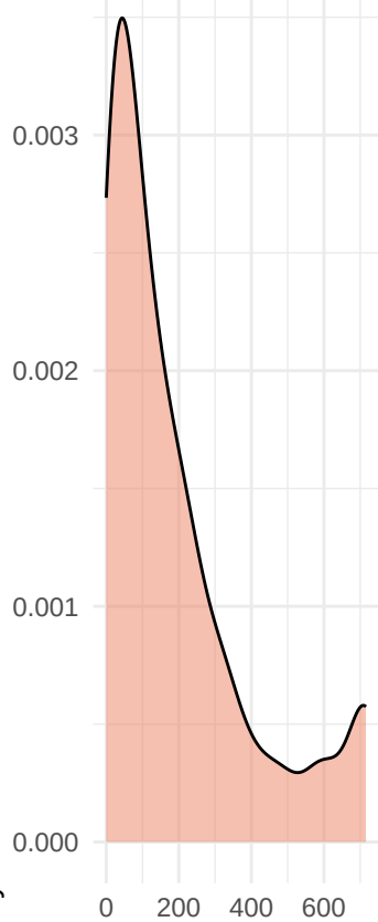
manganese
