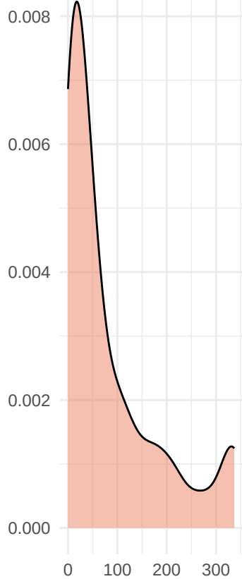
manganese
