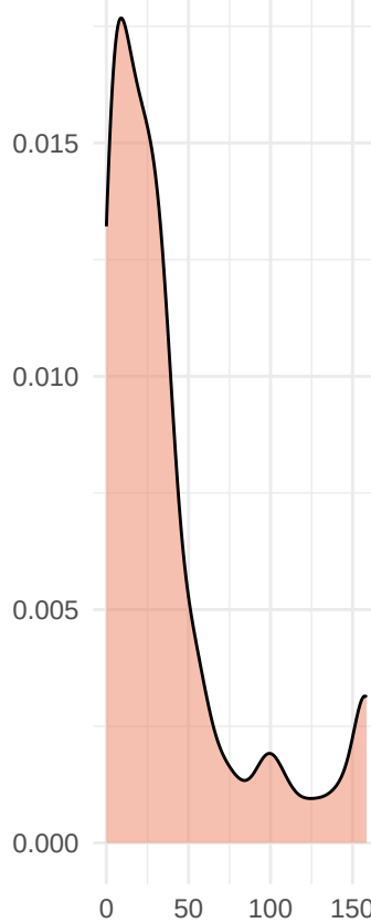
paraquats
