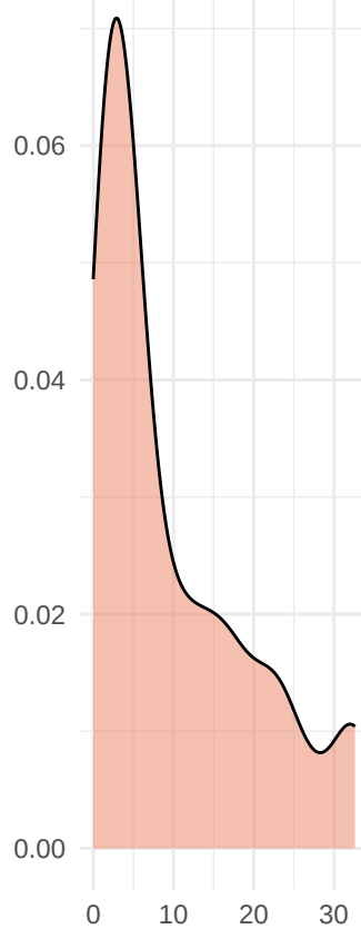
neonicotinoids
