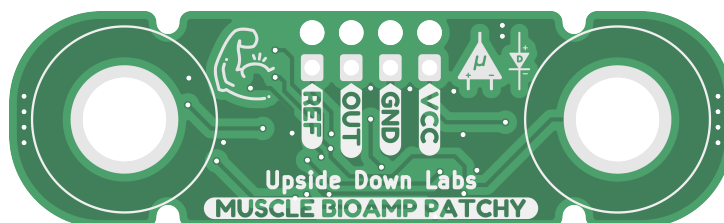
Fig. 2: PCB Back
