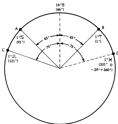
Figura 5. Una figura planetaria de cuatro factores (fórmula uraniana A + B - C = D ).
