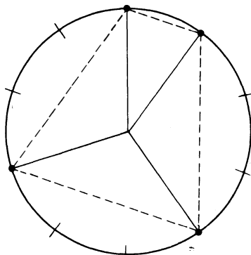
Una cadena de deciles
