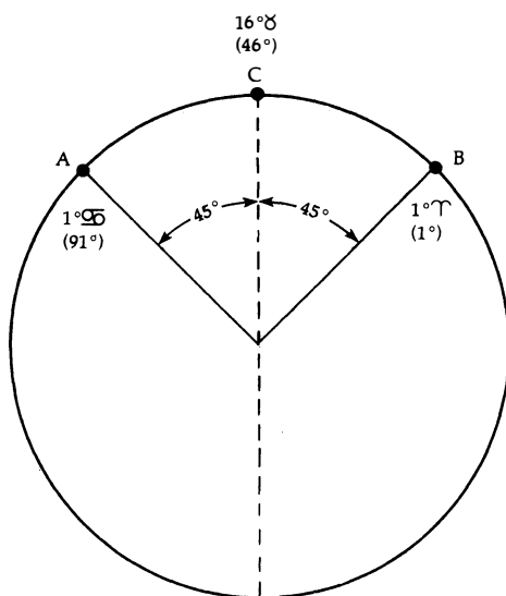
Figura 7. Un punto medio (fórmula uraniana A + B - C = C ).
