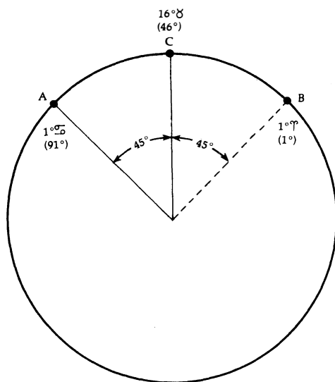
Figura 6. Una figura planetaria de tres factores (fórmula uraniana C + C - A = B ).
