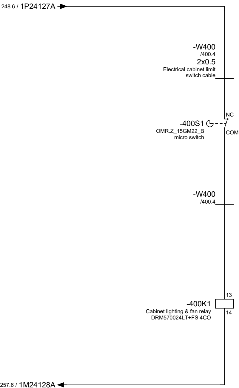
Cabinet light & fan control
