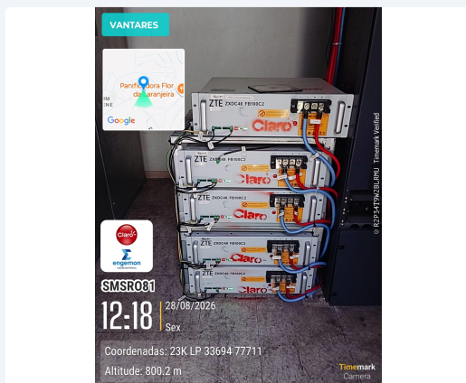
BATERIAS.jpeg
