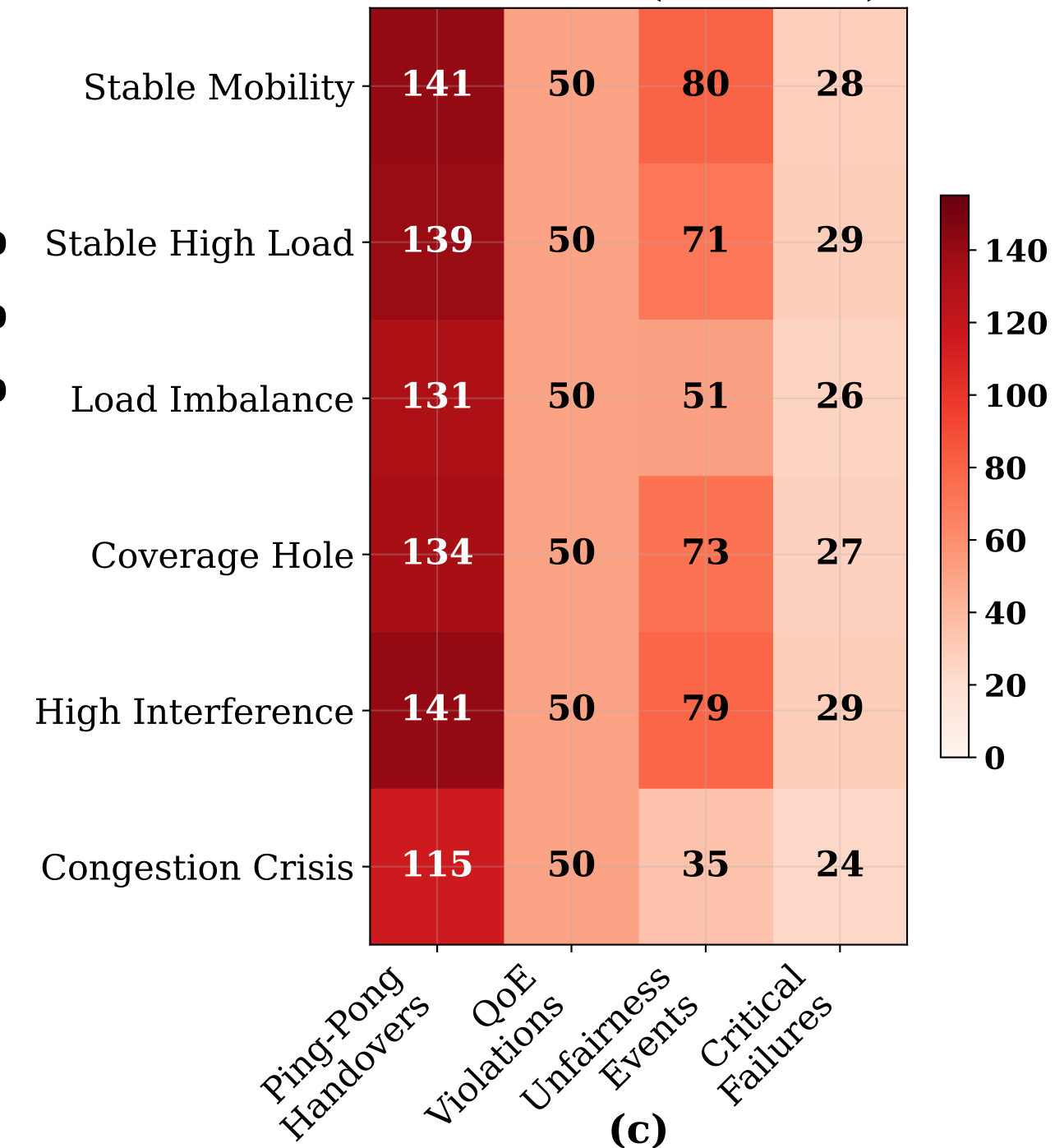
AI-Fuzzer (NSGA-II)
